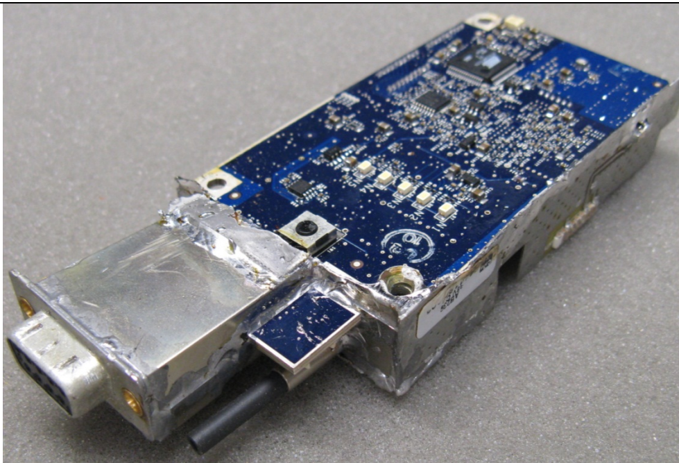
wSpO2 - Bottom of PCB
