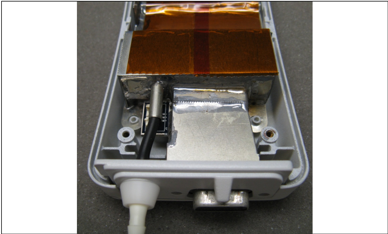
wSpO2 – Top (Zoomed In)
