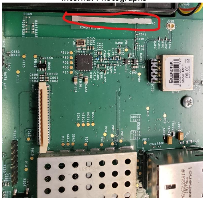
915 Antenna
