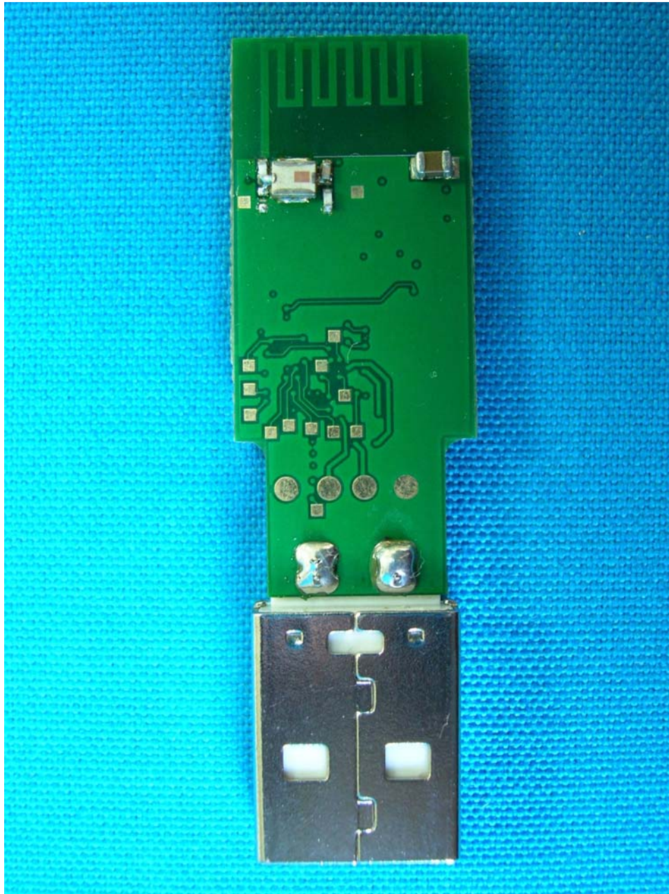
(17) EUT Photo
