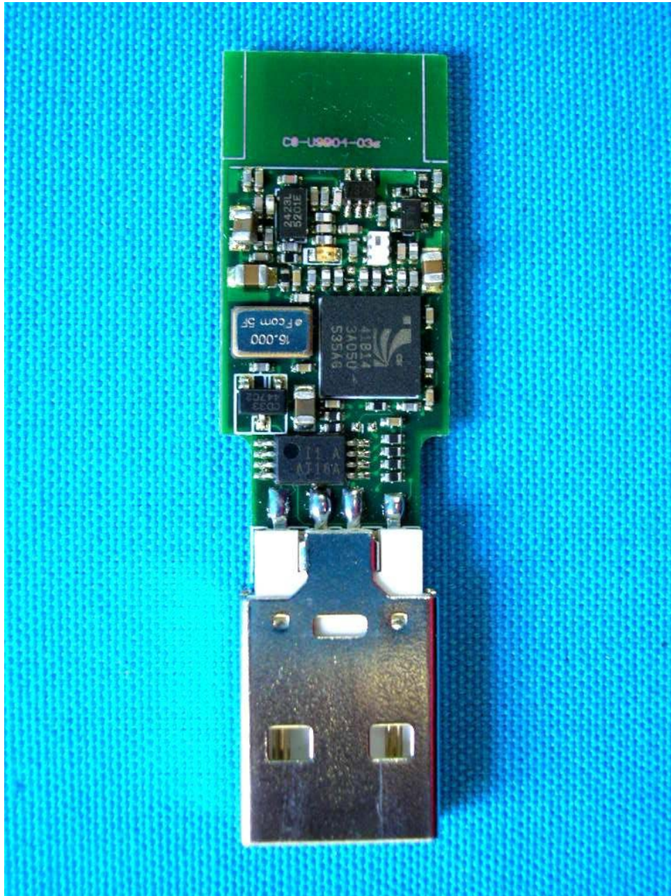
(16) EUT Photo
