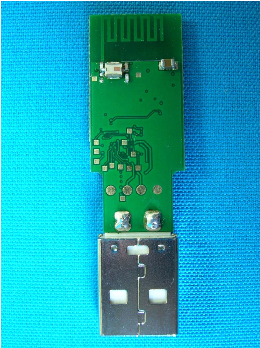
(5) EUT Photo
