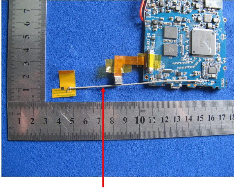
Antenna
