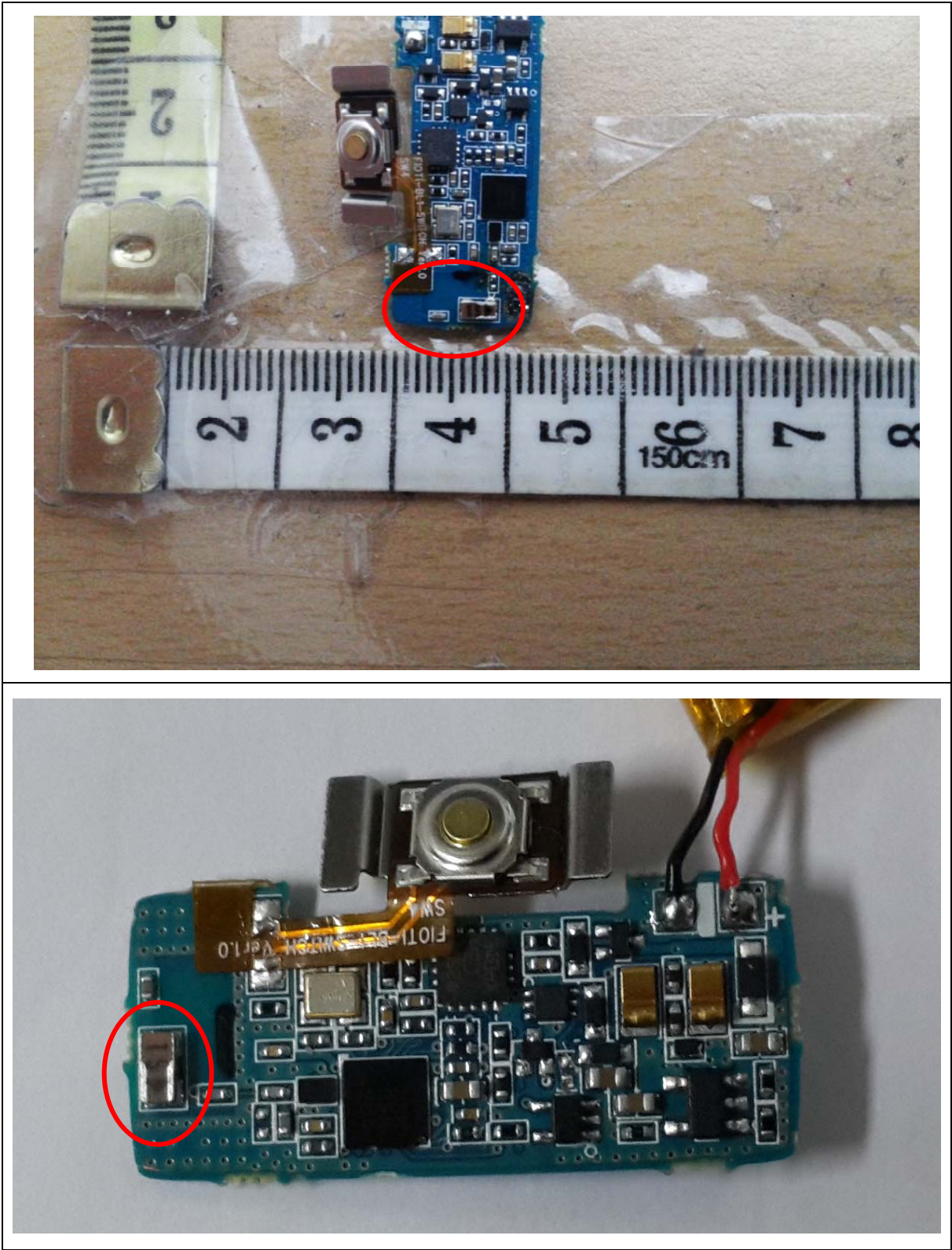
Antenna
