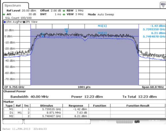
HT40 [Port 3]
