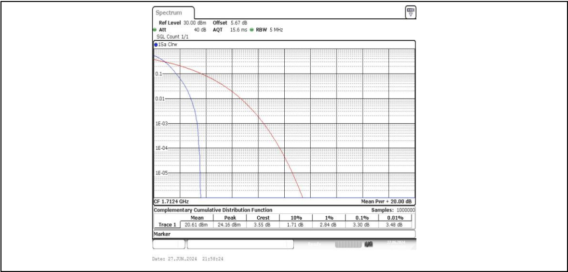
Band4-1312-1-PASS
