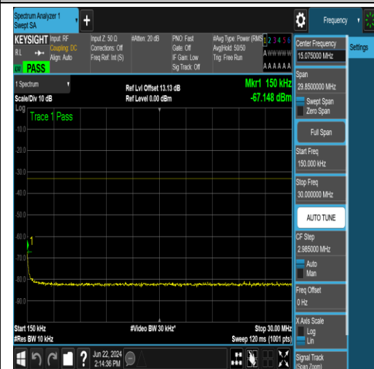
NTNV_N78-3700-3800_PC2_30_15_L_TID17_NS _01_1000_6000_#1
