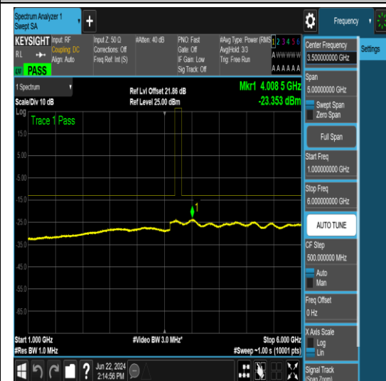
NTNV_N78-3700-3800_PC2_30_15_L_TID17_NS _01_18000_40000_#1
