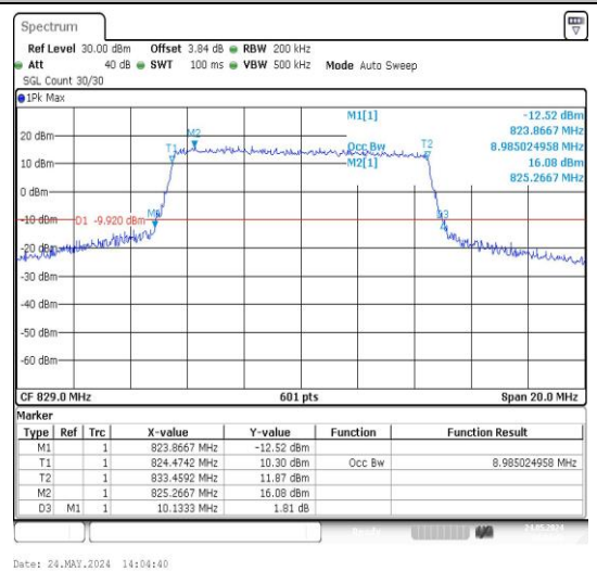
26(824-849)-10MHz-16QAM-26840-50RB#0-PASS
