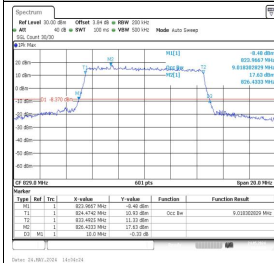
26(824-849)-10MHz-QPSK-26840-50RB#0-PASS
