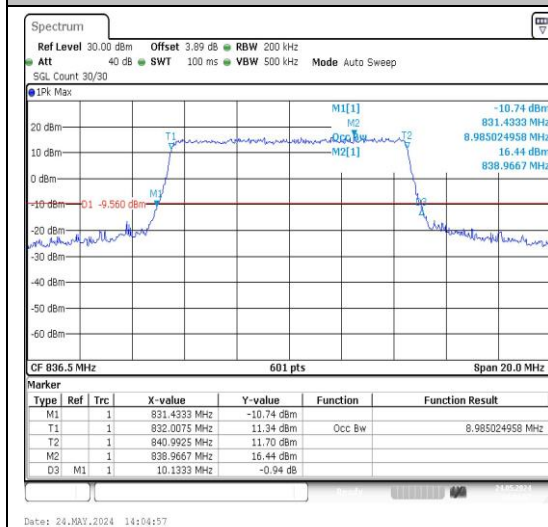
26(824-849)-10MHz-QPSK-26915-50RB#0-PASS
