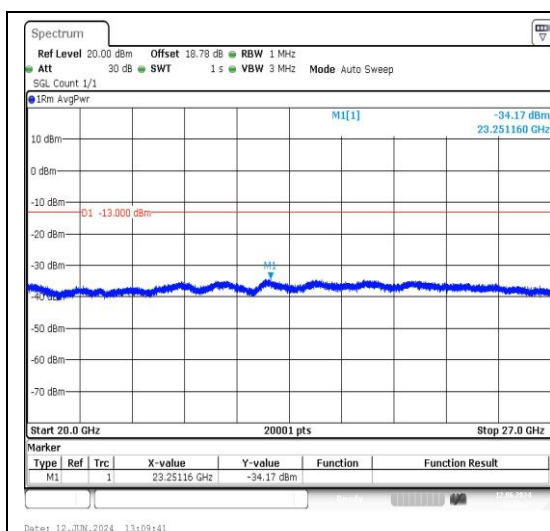
5-5-5MHz-10MHz-QPSK-QPSK-20428-20500-1R B#0-1RB#49-20000~27000MHz-PASS
