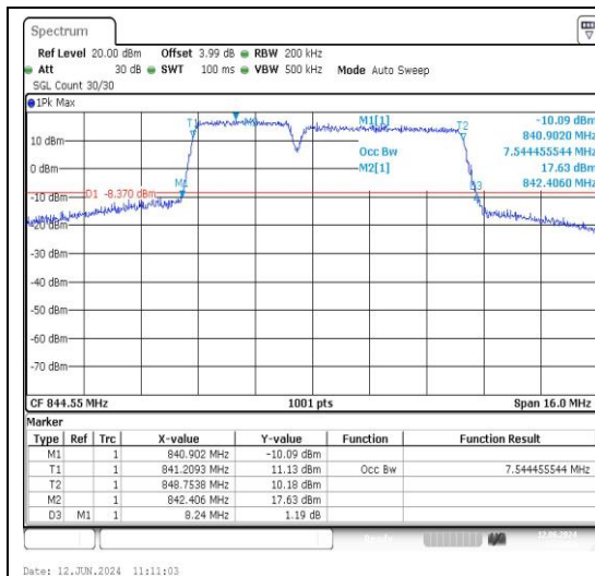
5-5-3MHz-5MHz-QPSK-QPSK-20586-20625-15R B#0-25RB#0-PASS
