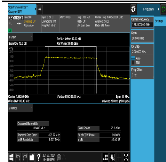
NTNV_DC_26A_n25A_PC3_15_5+10_M+M_TID1 _Ant1#1
