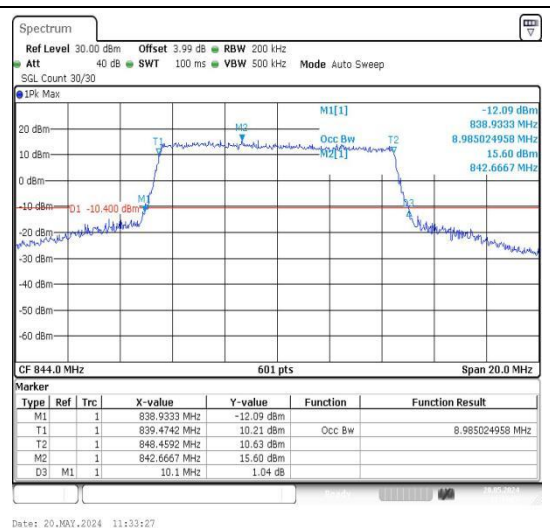
26(824-849)-10MHz-16QAM-26990-50RB#0-PASS
