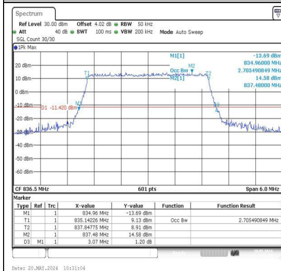
26(824-849)-3MHz-QPSK-26915-15RB#0-PASS
