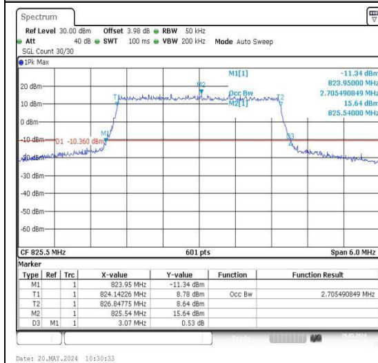
26(824-849)-3MHz-QPSK-26805-15RB#0-PASS
