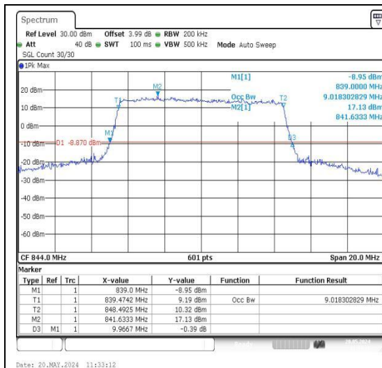
26(824-849)-10MHz-QPSK-26990-50RB#0-PASS
