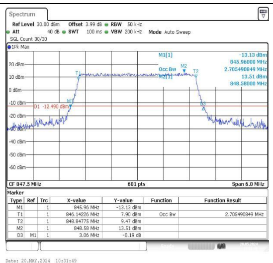
26(824-849)-3MHz-16QAM-27025-15RB#0-PASS
