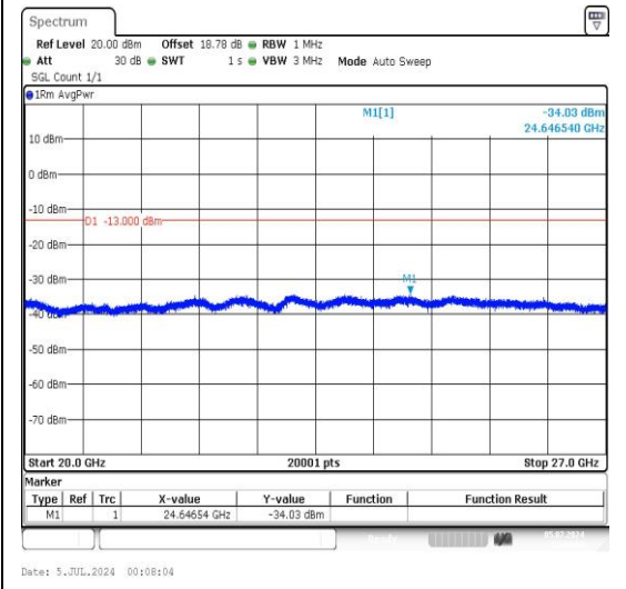
5-5-10MHz-5MHz-QPSK-QPSK-20550-20622-1R B#49-ORB#0-20000~27000MHz-PASS
