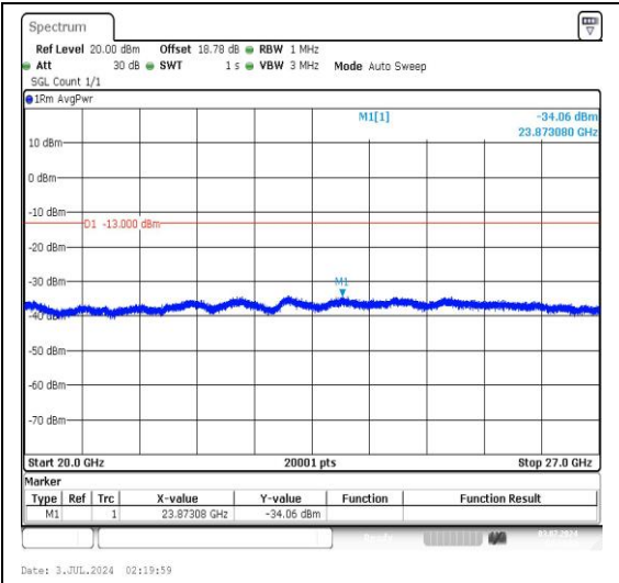
2-2-20MHz-5MHz-QPSK-QPSK-19050-19167-1R B#0-1RB#24-20000~27000MHz-PASS
