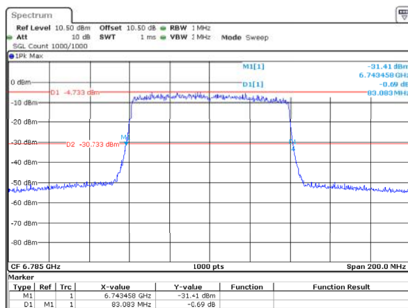
802.11ax80_6785MHz_RU_Full_ANT1 83.083MHz
