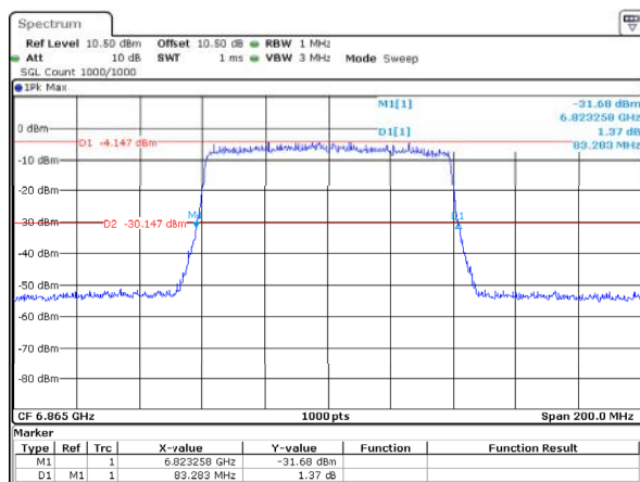
802.11ax80_6865MHz_RU_Full_ANT2 83.283MHz
