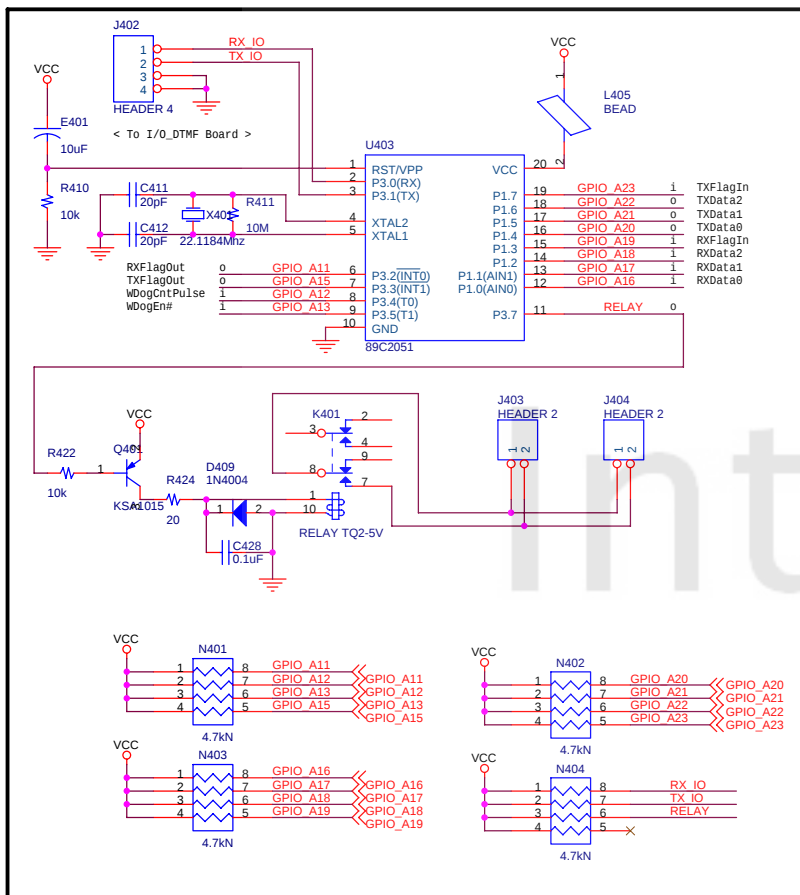
At89c2051 module
