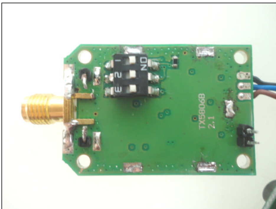
RF module
