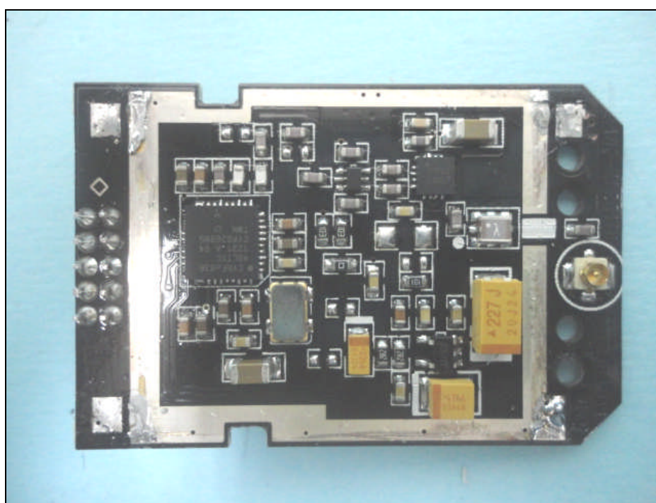
2.4 GHz DSSS Transceiver module
