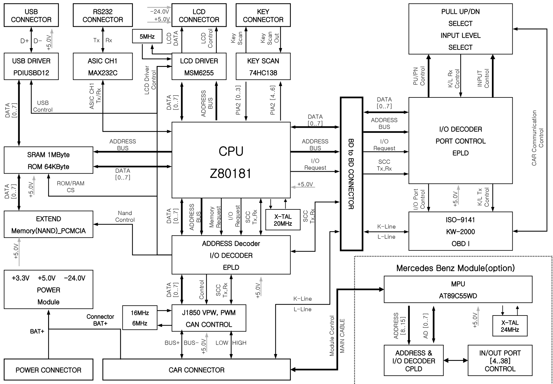
MULTISCAN plus Block Diagram(REV.3)
