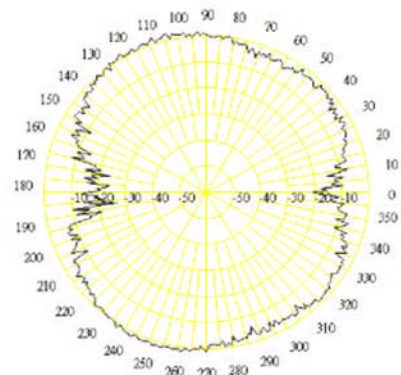
5.15~E-PLANE
