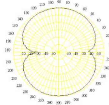
2.45-E-PLANE
