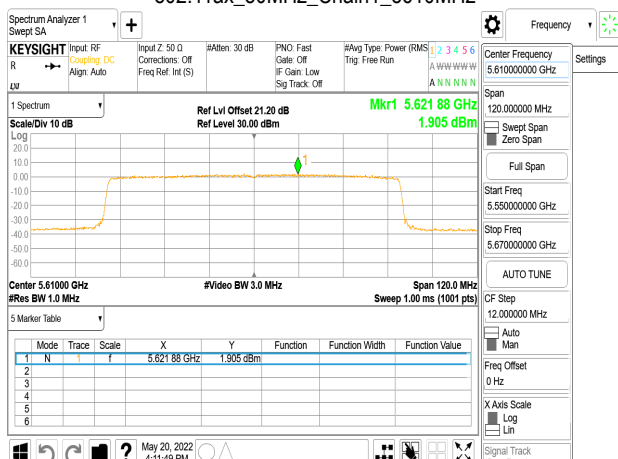
802.11ax_80MHz_Chain1_5610MHz_RU484_66
