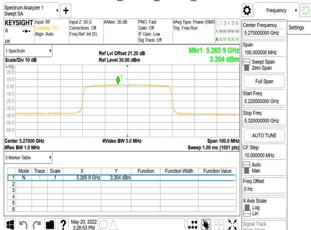
802.11ax_40MHz_Chain3_5270MHz
