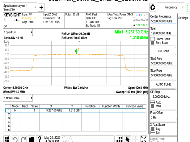
802.11ax_80MHz_Chain2_5290MHz_RU484_66
