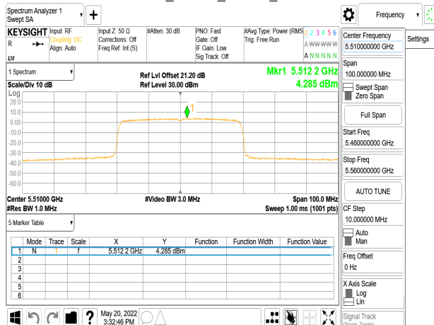
802.11ax_40MHz_Chain3_5510MHz
