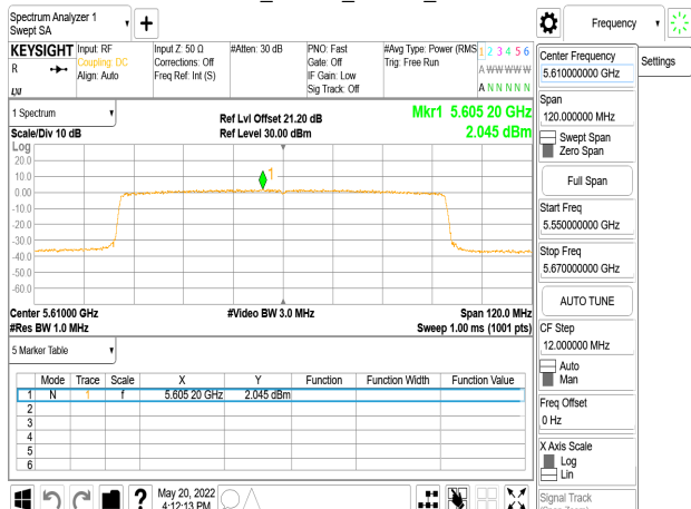
802.11ax_80MHz_Chain2_5610MHz
