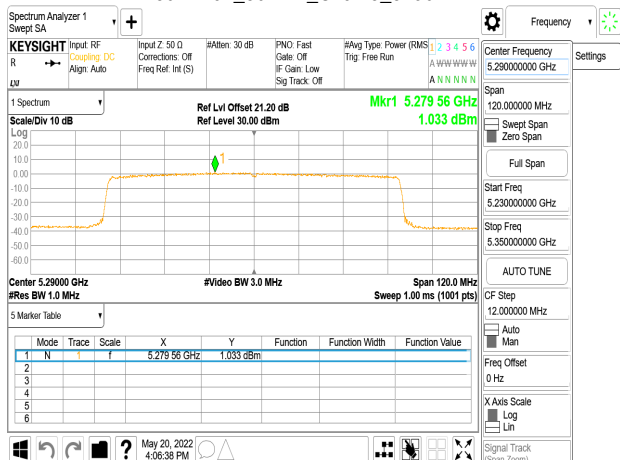
802.11ax_80MHz_Chain3_5290MHz_RU484_66
