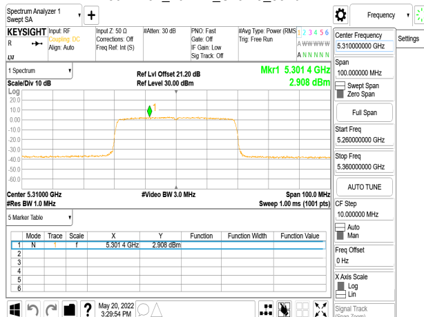
802.11ax_40MHz_Chain3_5310MHz_RU242_62
