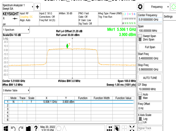
802.11ax_40MHz_Chain2_5510MHz_RU242_61
