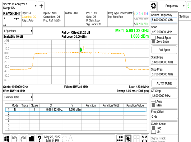
802.11ax_80MHz_Chain2_5690MHz_UNII_3
