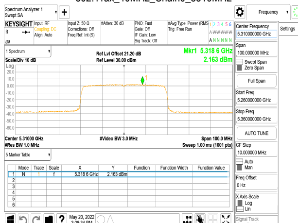
802.11ax_40MHz_Chain0_5310MHz_RU242_62
