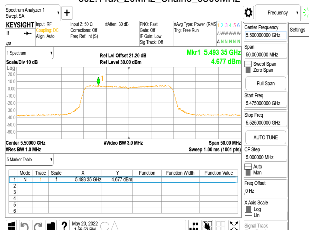
802.11ax_20MHz_Chain3_5500MHz_RU106_53
