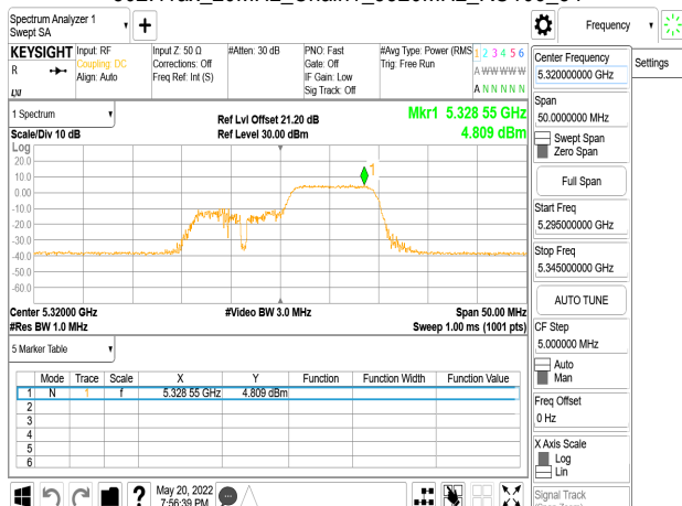
802.11ax_20MHz_Chain1_5320MHz_RU106_54
