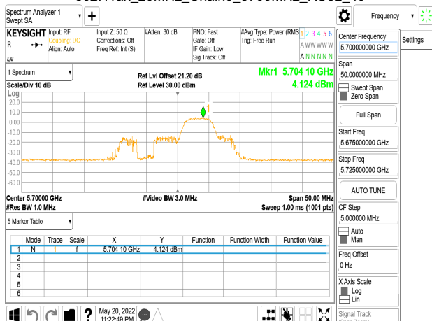
802.11ax_20MHz_Chain0_5700MHz_RU52_40
