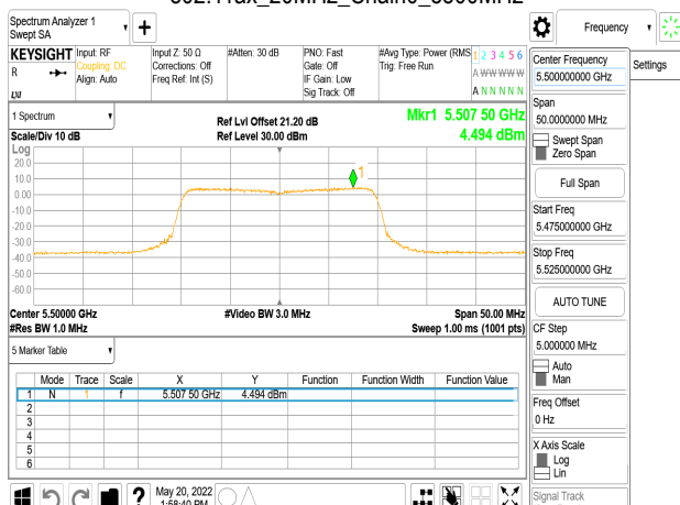
802.11ax_20MHz_Chain0_5500MHz_RU106_53
