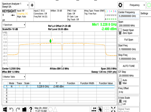
802.11ac_160MHz_Chain2_5250MHz
