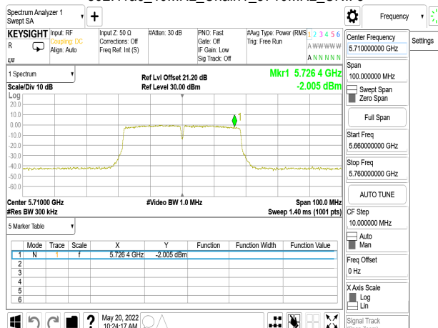
802.11ac_40MHz_Chain1_5710MHz_UNII 3
