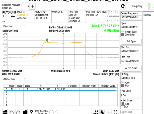
802.11ac_20MHz_Chain2_5720MHz_UNII 3
