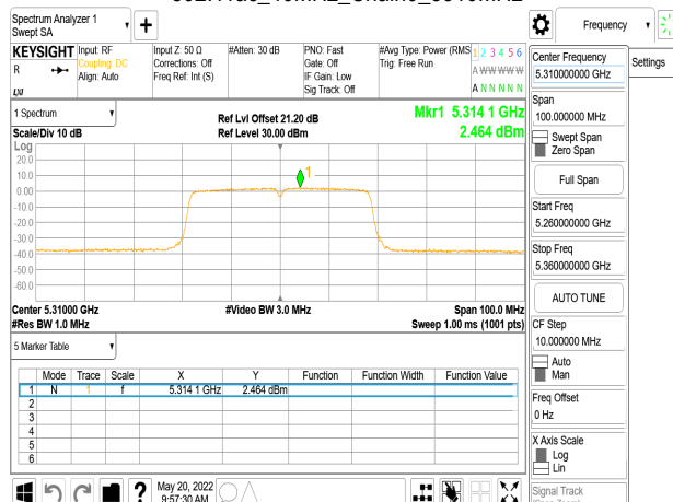
802.11ac_40MHz_Chain0_5310MHz
