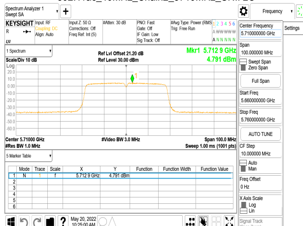
802.11ac_40MHz_Chain2_5710MHz_UNII 2C
