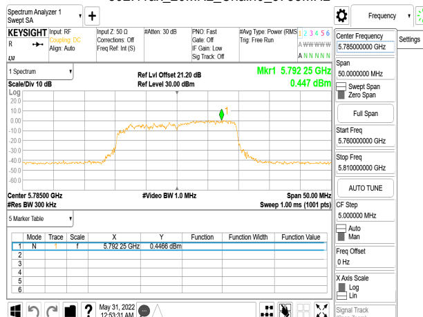
802.11ax_20MHz_Chain0_5785MHz
