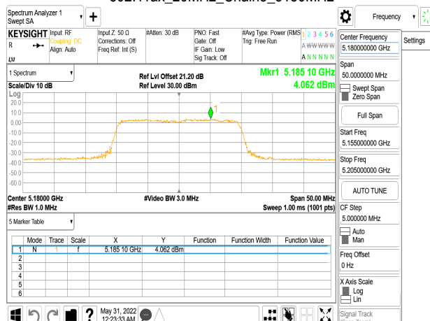
802.11ax_20MHz_Chain3_5180MHz_RU106_53
