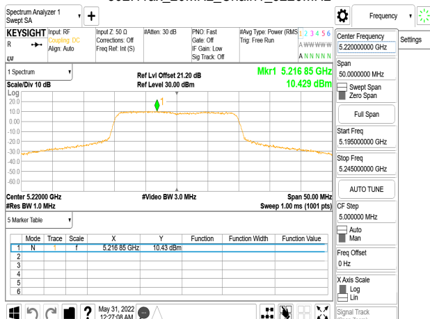
802.11ax_20MHz_Chain1_5220MHz
