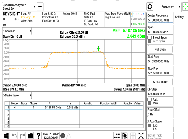
802.11ax_20MHz_Chain2_5180MHz_RU106_53
