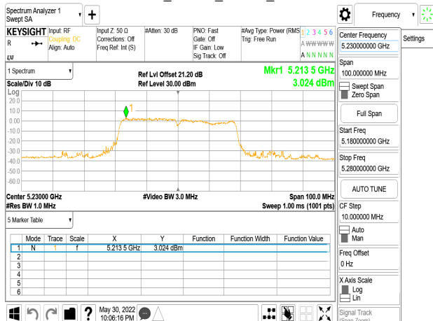
802.11ac_40MHz_Chain3_5230MHz
