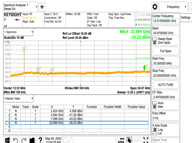
802.11n_40MHz_Chain1_2437MHz
