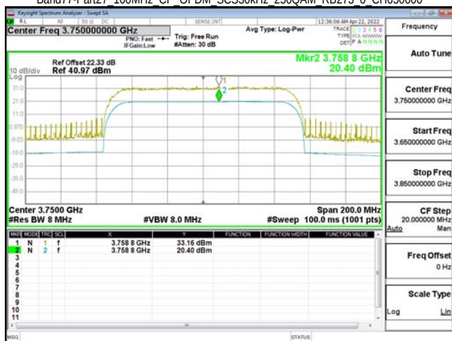
Band77-Part27 100MHz CP OFDM SCS30kHz 256QAM RB273 0 CH650000
