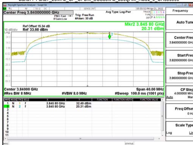
Band77-Part27 20MHz CP OFDM SCS30kHz 256QAM RB51 0 CH656000
