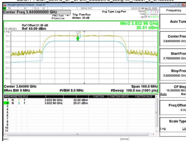
Band77-Part27 80MHz CP OFDM SCS30kHz 256QAM RB217 0 CH656000
