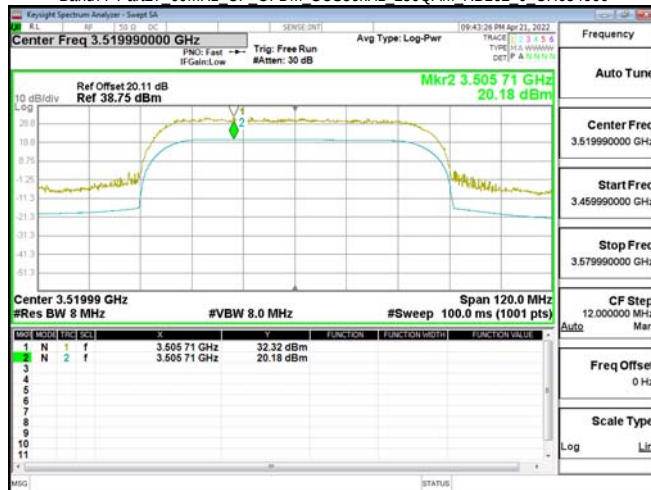
Band77-Part27 60MHz CP OFDM SCS30kHz 256QAM RB162 0 CH634666
