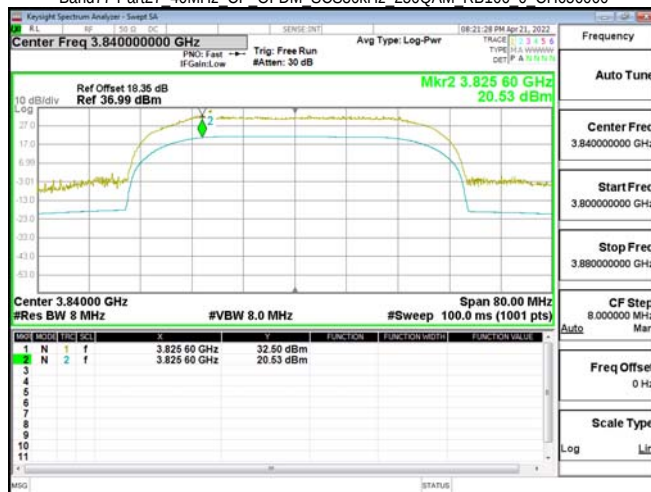
Band77-Part27 40MHz CP OFDM SCS30kHz 256QAM RB106 0 CH656000
