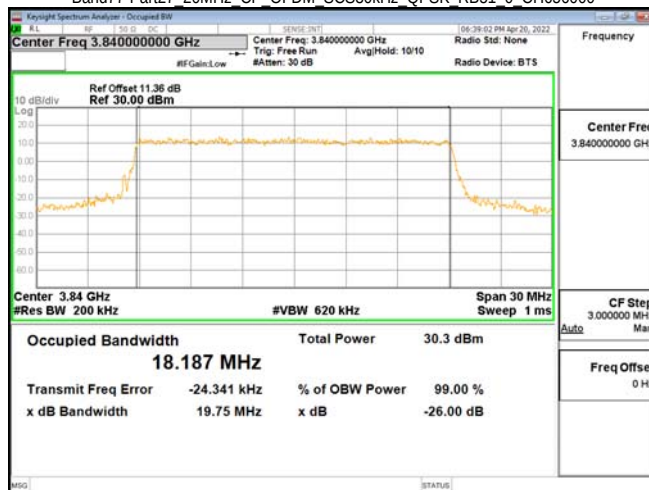
Band77-Part27 20MHz CP OFDM SCS30kHz QPSK RB51 0 CH656000
