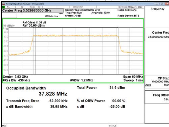
Band77-Part27 40MHz CP OFDM SCS30kHz QPSK RB106 0 CH635332
