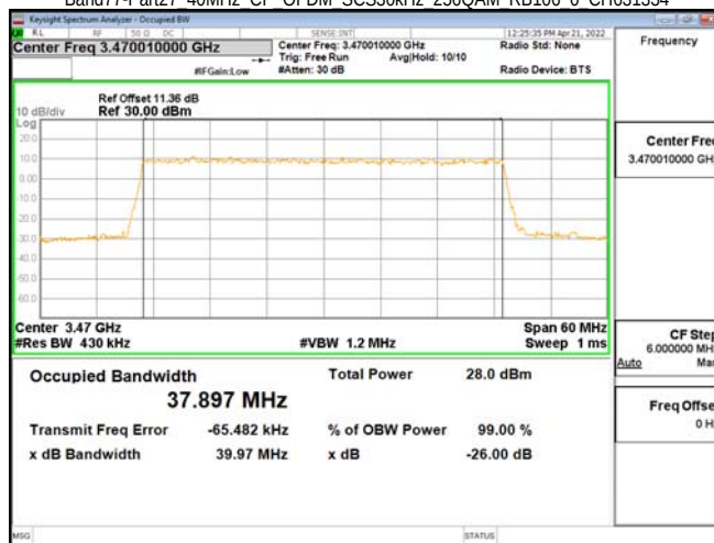
Band77-Part27 40MHz CP OFDM SCS30kHz 256QAM RB106 0 CH633334
