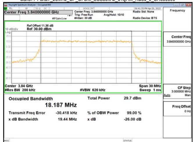
Band77-Part27 20MHz CP OFDM SCS30kHz 64QAM RB51 0 CH656000
