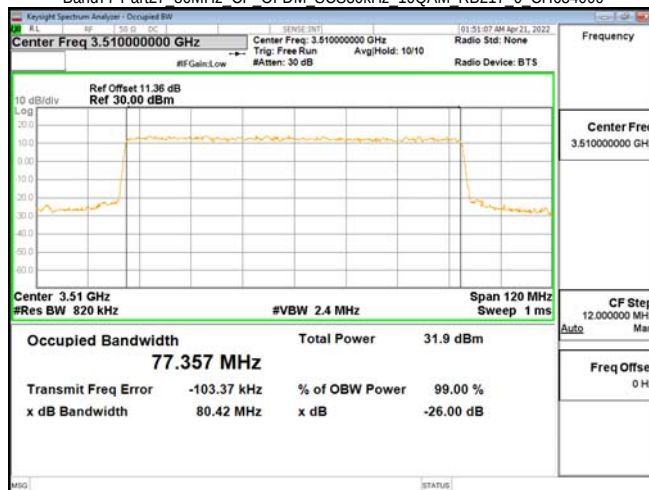
Band77-Part27 80MHz CP OFDM SCS30kHz 16QAM RB217 0 CH634000
