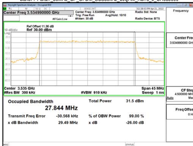
Band77-Part27 30MHz CP OFDM SCS30kHz 16QAM RB78 0 CH635666
