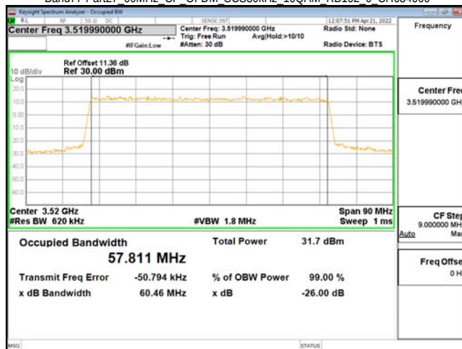
Band77-Part27 60MHz CP OFDM SCS30kHz 16QAM RB162 0 CH634666
