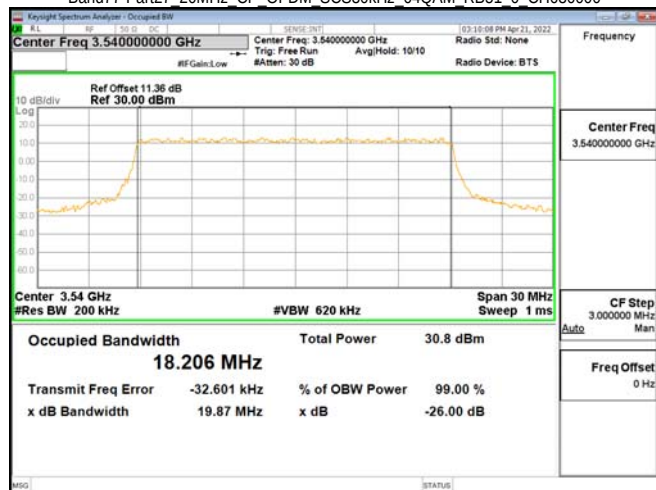
Band77-Part27 20MHz CP OFDM SCS30kHz 64QAM RB51 0 CH636000
