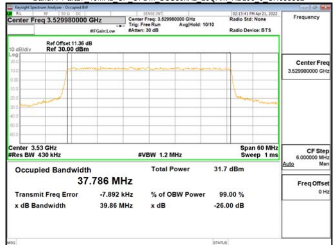
Band77-Part27 40MHz CP OFDM SCS30kHz 16QAM RB106 0 CH635332
