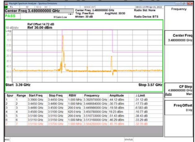
Band77-Part27 60MHz DFT s OFDM SCS30kHz BPSK RB1 0 CH633334
