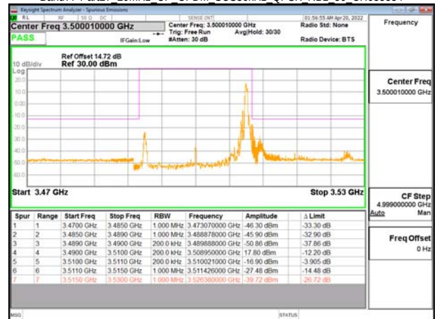
Band77-Part27 20MHz CP OFDM SCS30kHz QPSK RB1 50 CH633334
