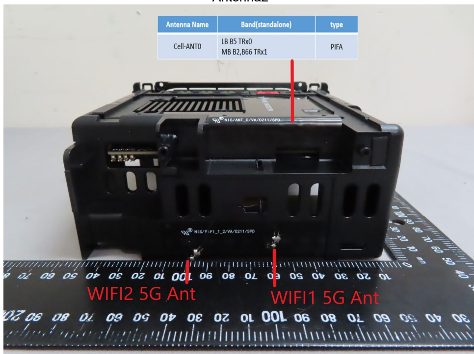
Antenna2
