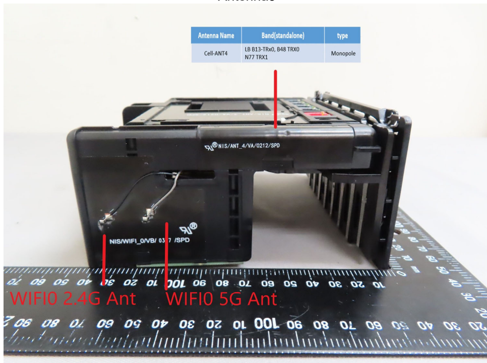
Antenna4
