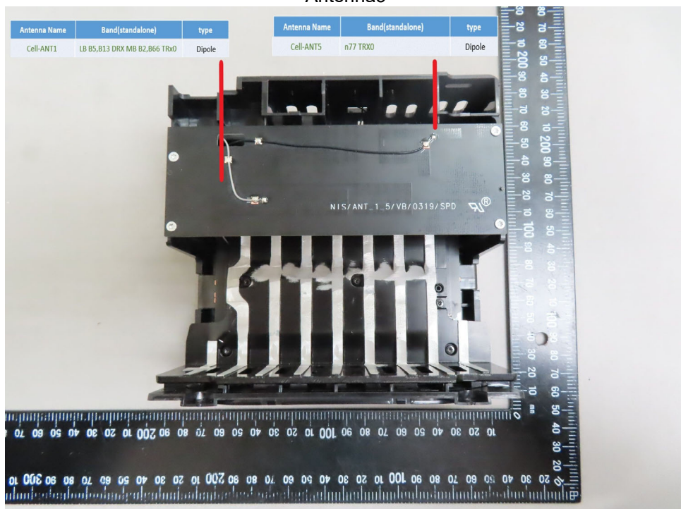
Antenna5
