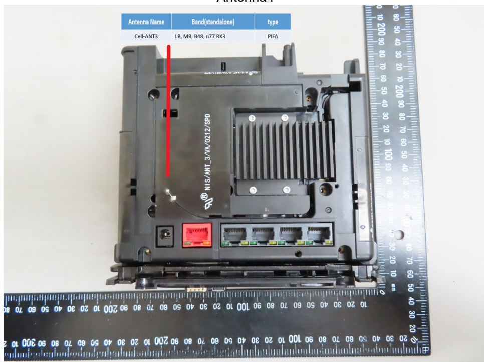
Antenna4
