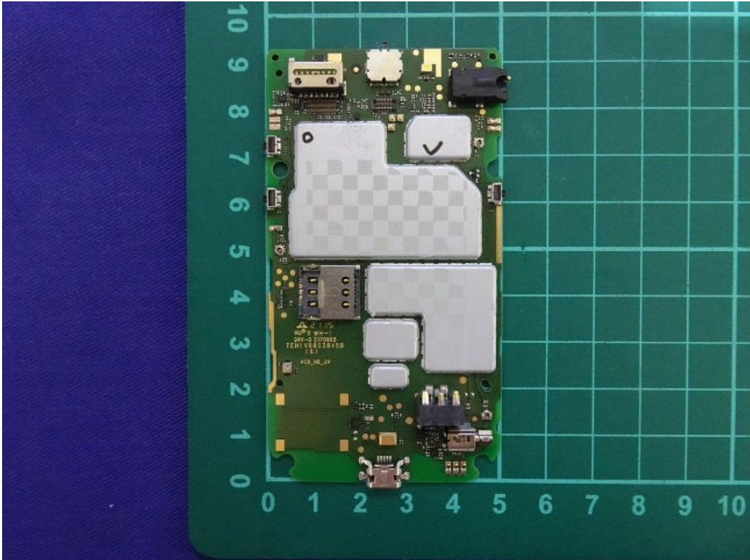
(24) EUT Photo
