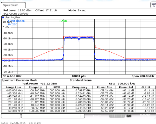
NTNV-11AX40MIMO-Ant1-6685-PASS
