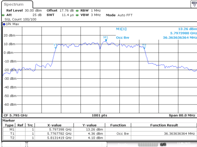
11N40MIMO-Ant2-5795
