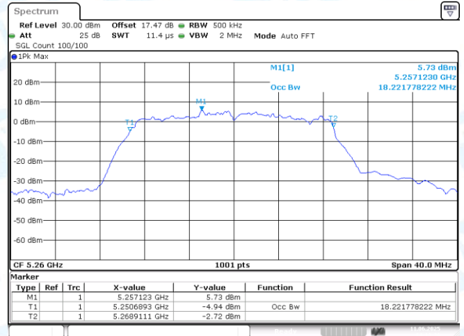
11AC20MIMO-Ant1-5260
