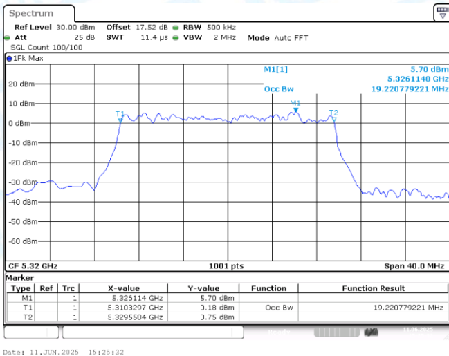
11AX20MIMO-Ant2-5320
