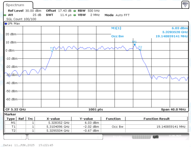
11AX20MIMO-Ant1-5320
