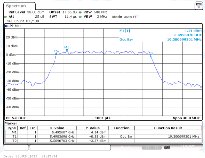
11AX20MIMO-Ant1-5500
