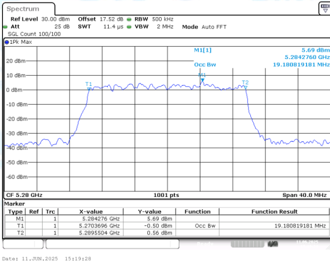
11AX20MIMO-Ant2-5280
