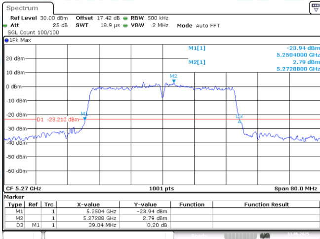
11AC40MIMO-Ant1-5270
