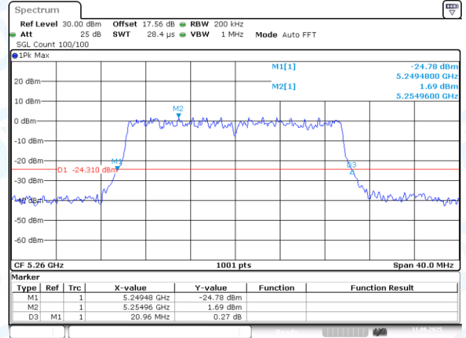
11AX20MIMO-Ant2-5260
