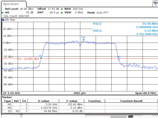
11AC40MIMO-Ant1-5550
