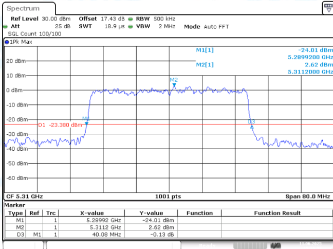
11AX40MIMO-Ant1-5310
