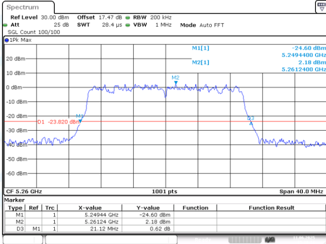
11AX20MIMO-Ant1-5260
