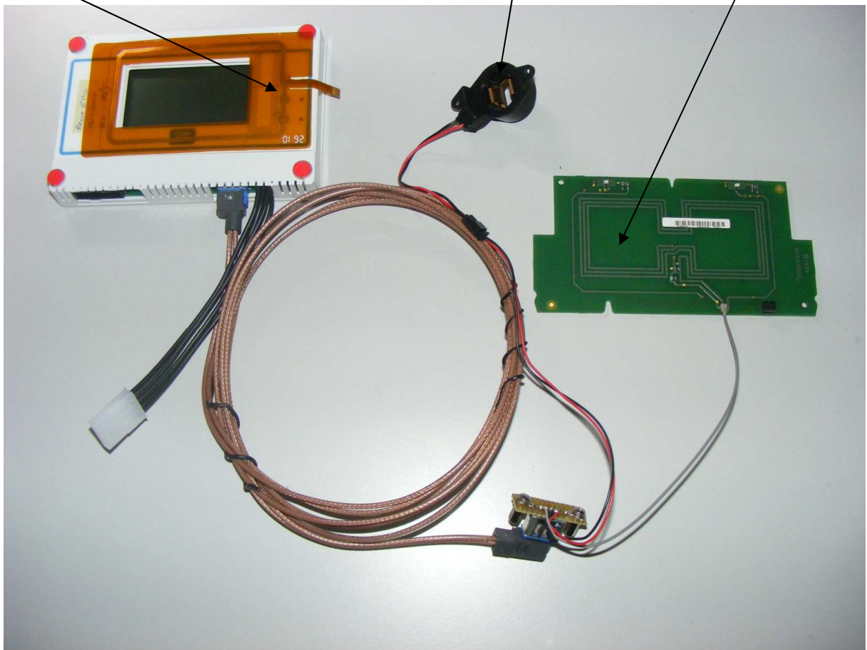
RFID 1 Antenna (Build in)t
