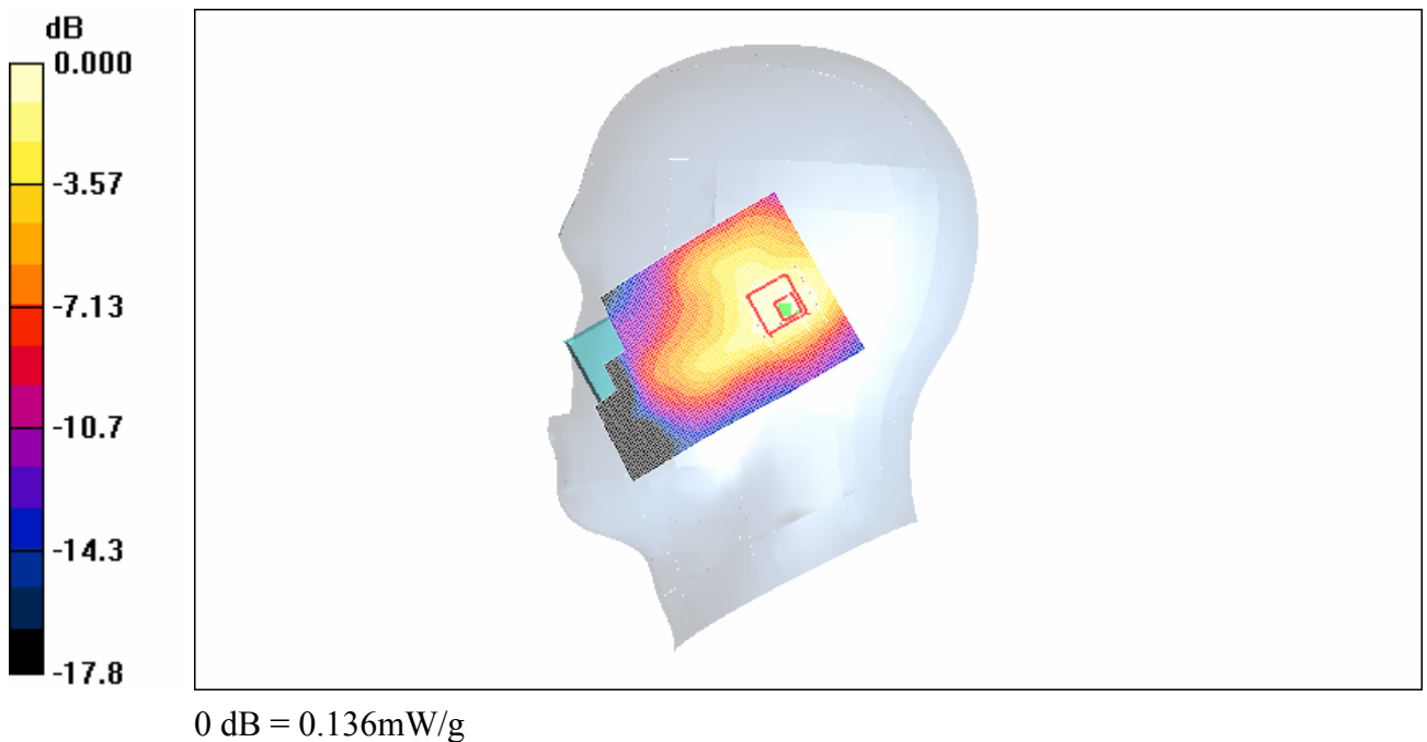
Fig. 15 1900 MHz CH661
