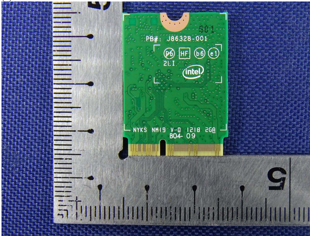
(2) EUT Photo
