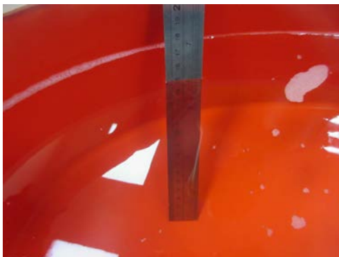
Body(2450MHz)_15.1cm
