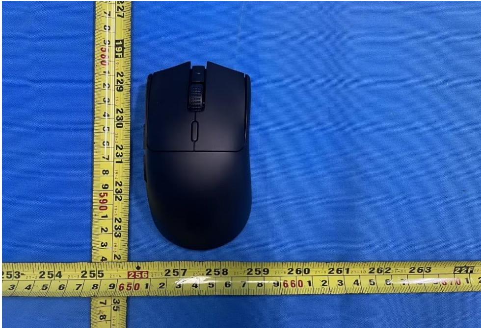
(6) EUT Photo
