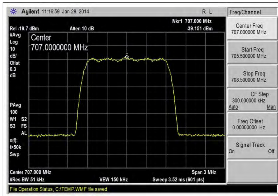
CDMA_UL 698-716_Input
