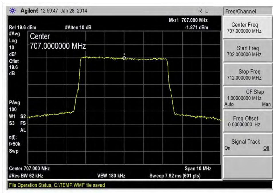
LTE_UL 698-716_Output
