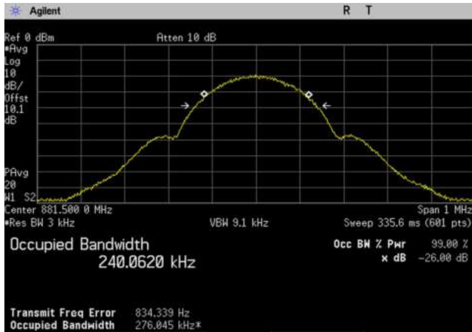
7.10 OBW-Out_DL_869-894_GSM_ 881.5MHz
