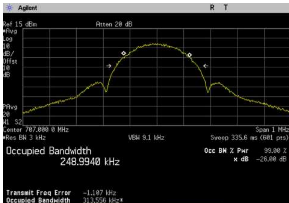
7.10 OBW-Out_UL_698-716_EDGE_707MHz
