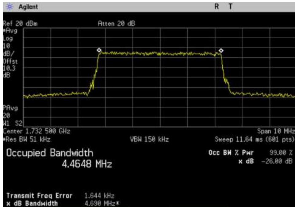
7.10 OBW-Out_UL_1710-1755_LTE_1732.5MHz
