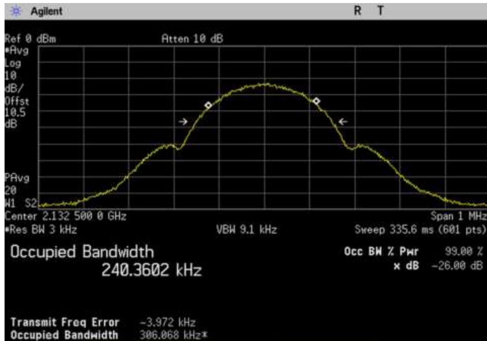
7.10 OBW-Out_DL_2110-2155_GSM_ 2132.5MHz
