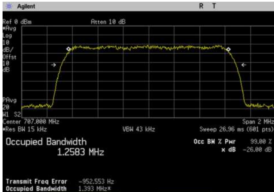
7.10 OBW-In_UL_698-716_CDMA_ 707MHz
