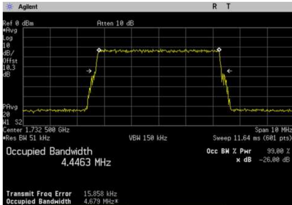
7.10 OBW-In_UL_1710-1755_LTE_ 1732.5MHz
