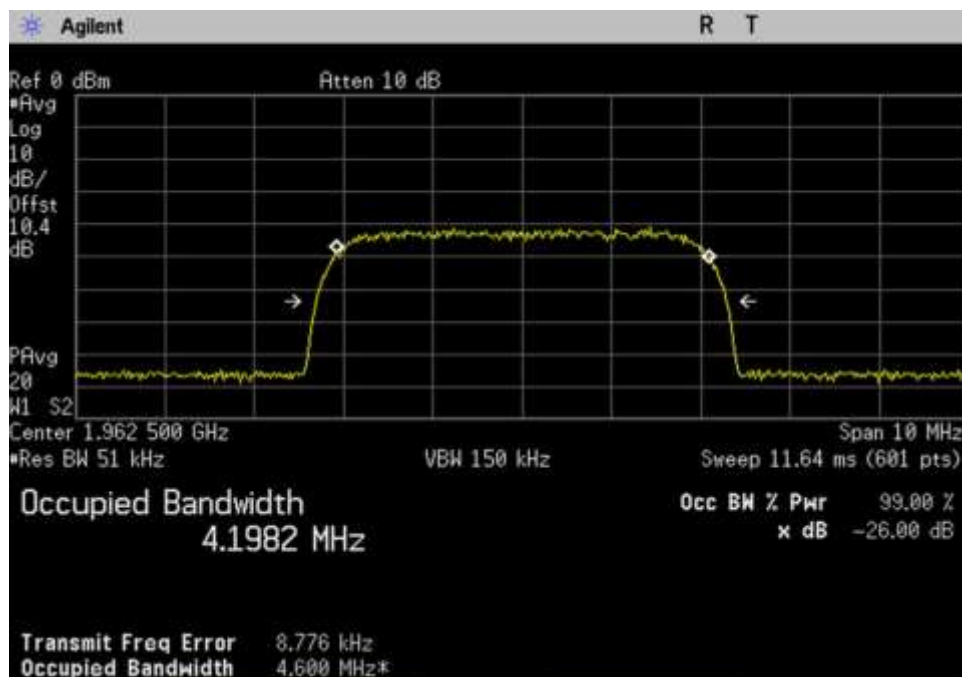
7.10 OBW-In_DL_1930-1995_WCDMA_1962.5MHz
