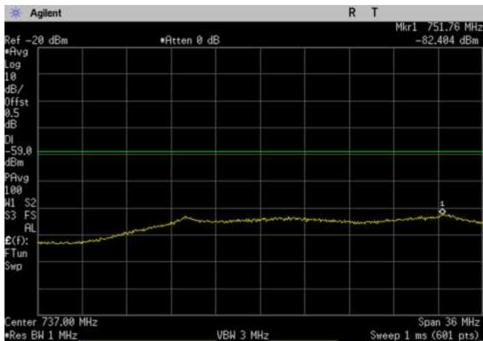
7.7 Noise_DL_728-746_ 737MHz
