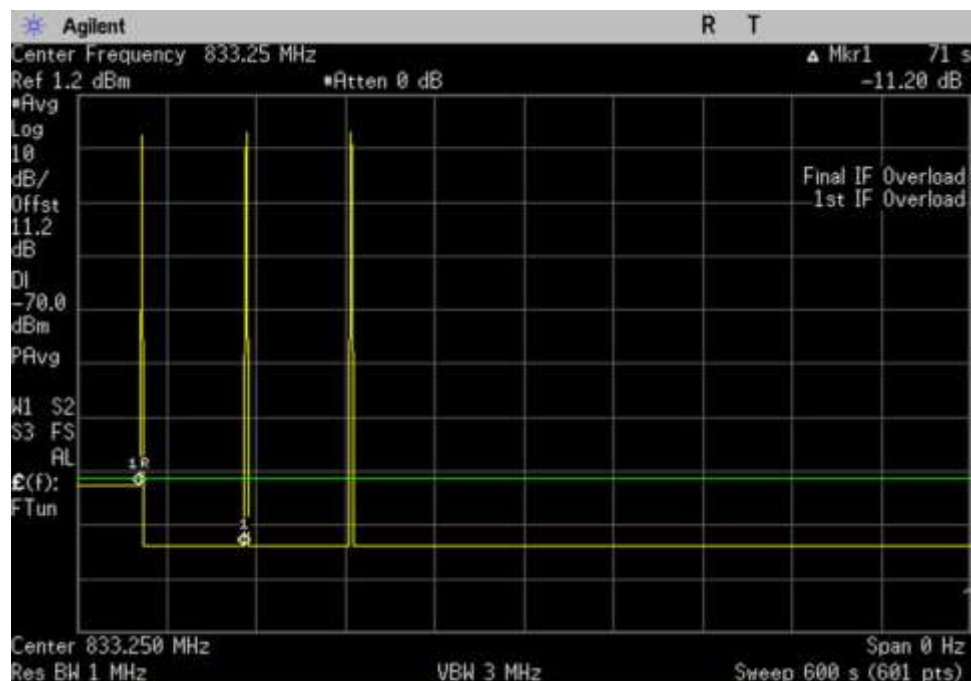
7.11.2 Osc_UL_824-849_600sec_ 833.25MHz
