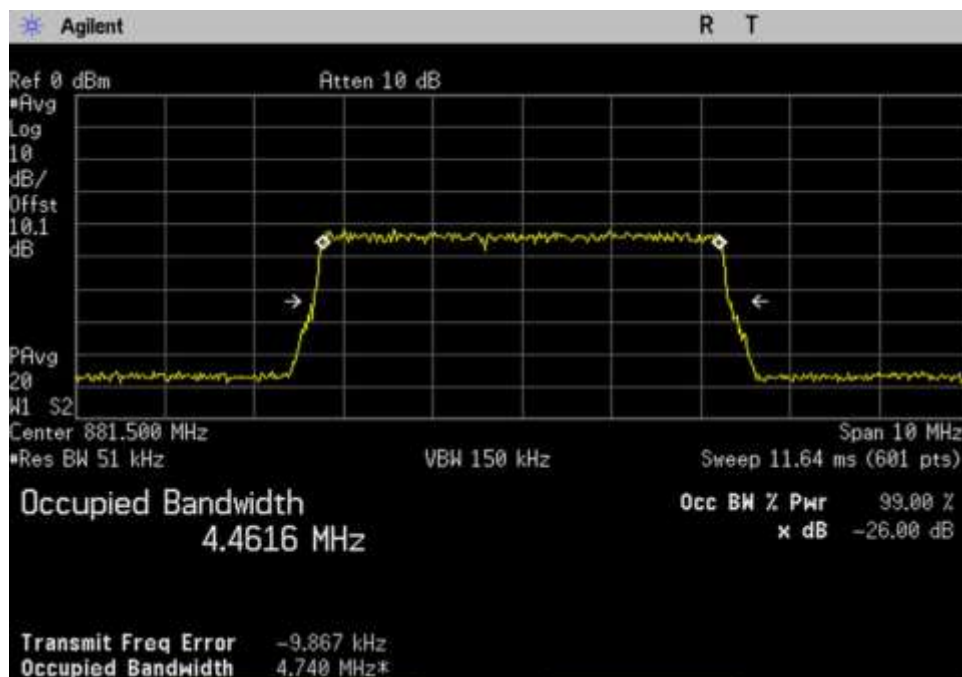
7.10 OBW-In_DL_869-894_LTE_ 881.5MHz
