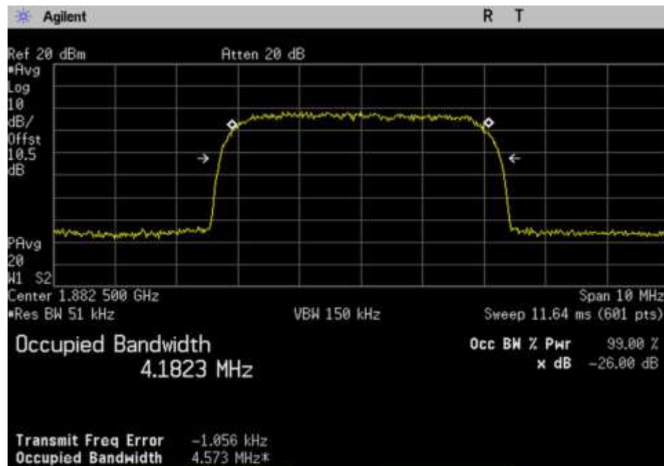
7.10 OBW-Out_UL_1850-1915_WCDMA_1882.5MHz
