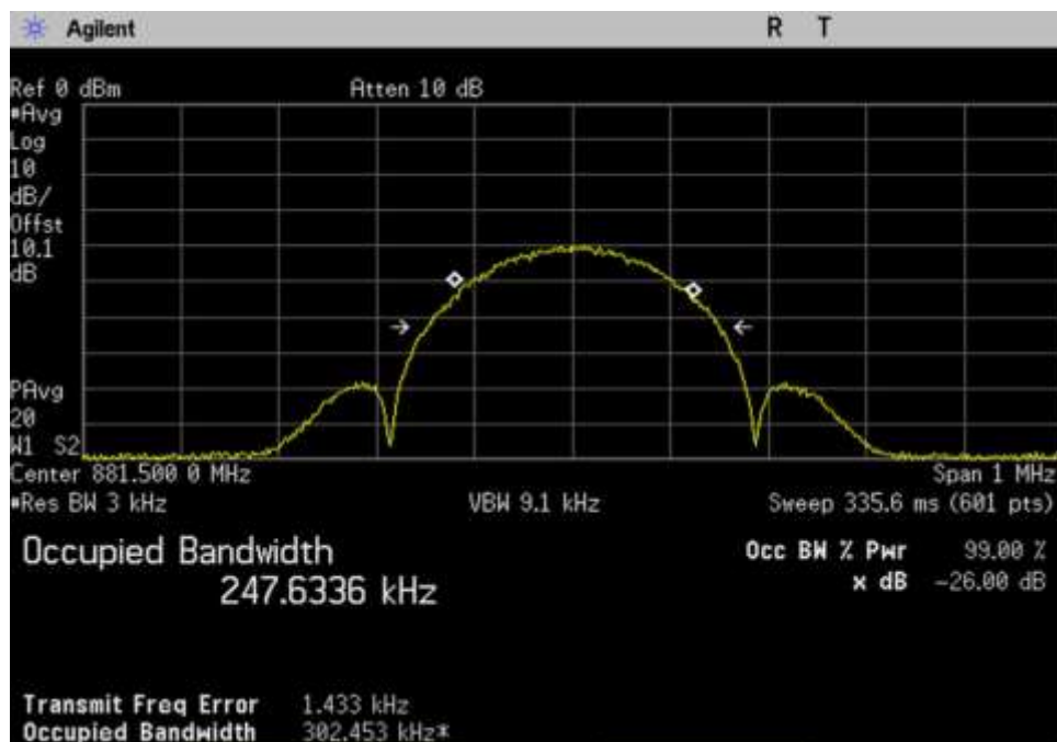
7.10 OBW-In_DL_869-894_EDGE_ 881.5MHz
