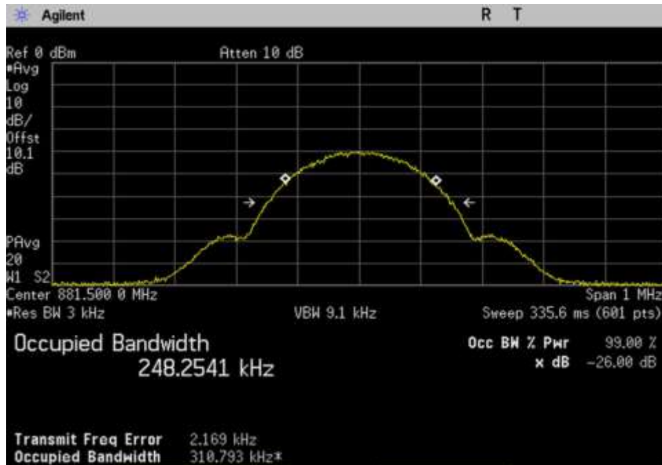
7.10 OBW-In_DL_869-894_GSM_ 881.5MHz
