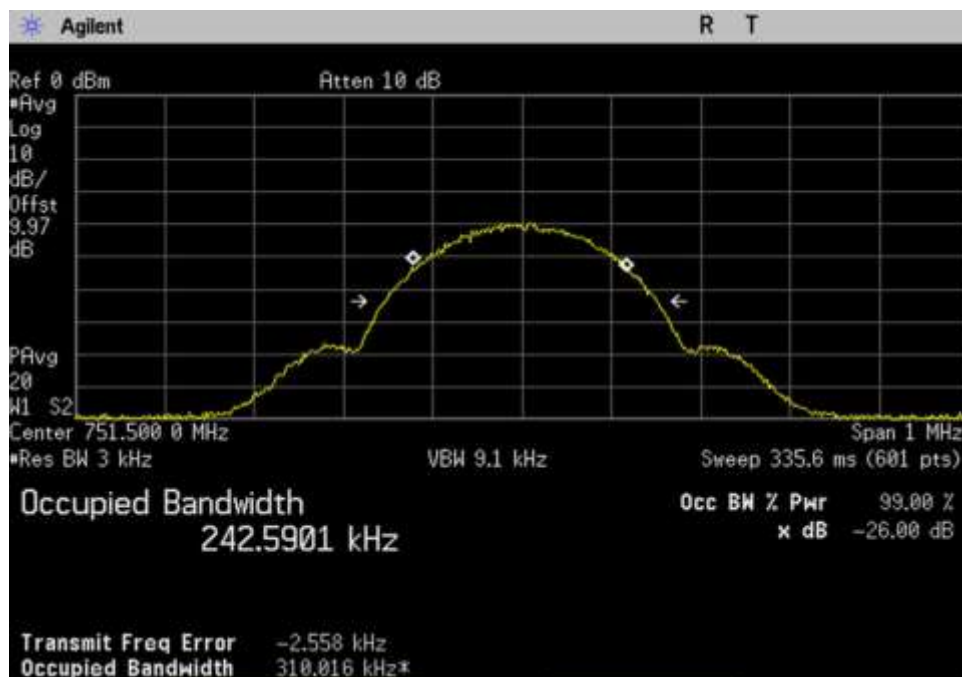
7.10 OBW-In_DL_746-757_GSM_ 751.5MHz
