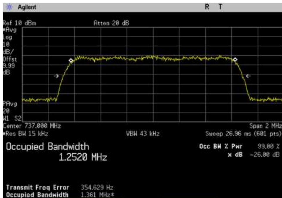
7.10 OBW-Out_DL_728-746_CDMA_737MHz
