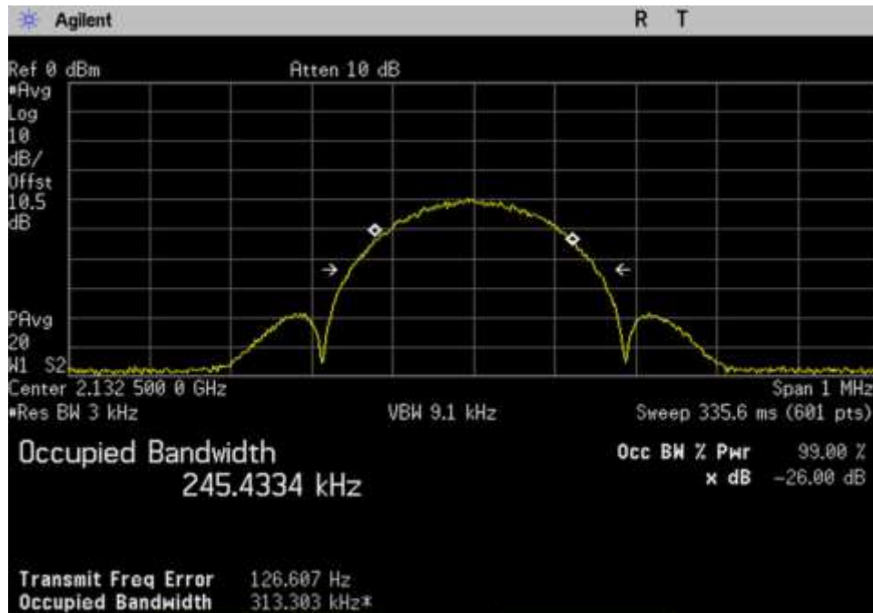
7.10 OBW-In_DL_2110-2155_GSM_ 2132.5MHz
