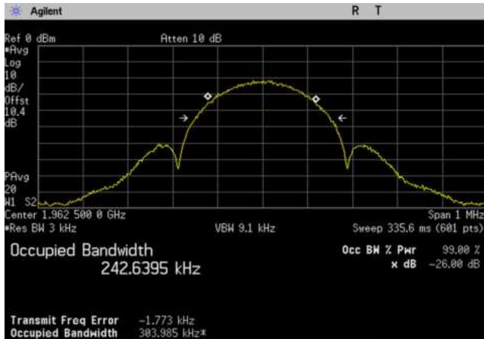
7.10 OBW-Out_DL_1930-1995_EDGE_ 1962.5MHz
