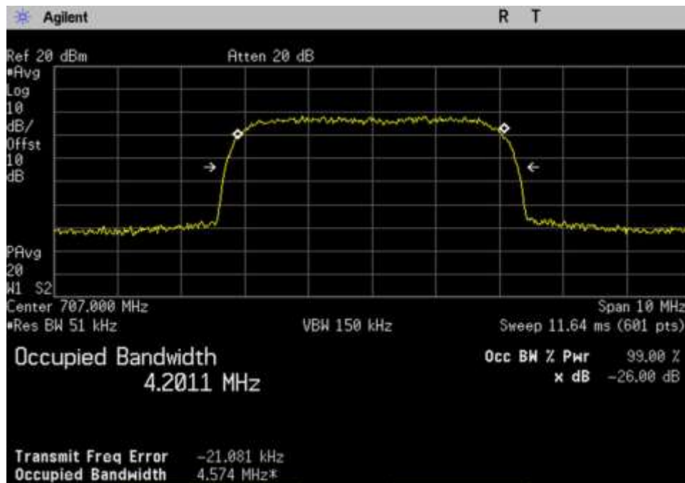
7.10 OBW-Out_UL_698-716_WCDMA_707MHz
