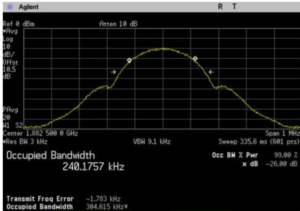
7.10 OBW-In_UL_1850-1915_GSM_ 1882.5MHz
