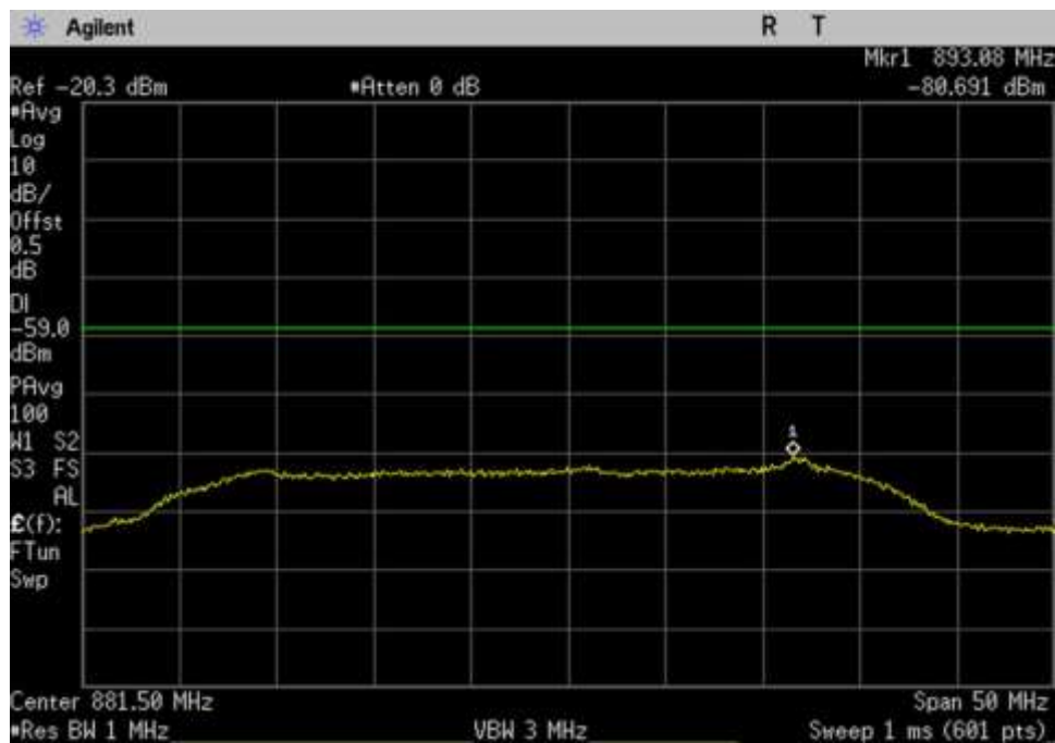
7.7 Noise_DL_869-894_ 881.5MHz
