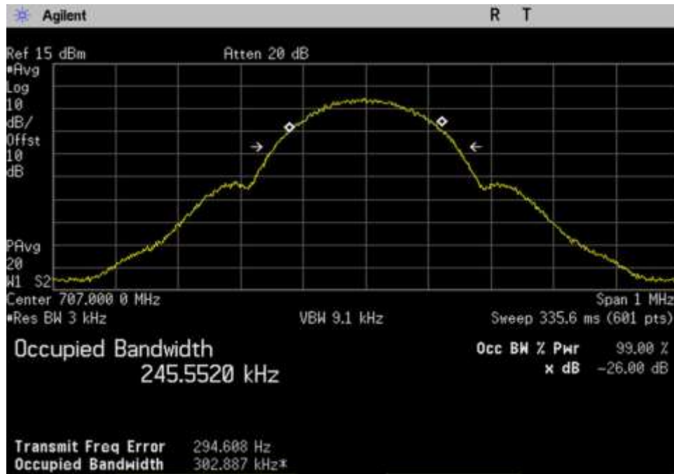
7.10 OBW-Out_UL_698-716_GSM_ 707MHz
