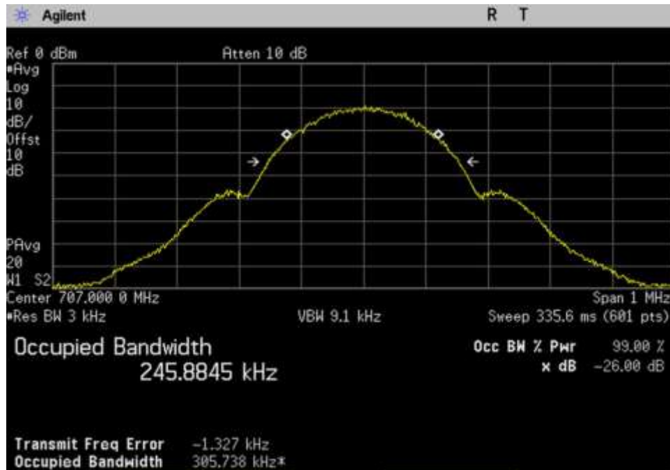
7.10 OBW-In_UL_698-716_GSM_707MHz
