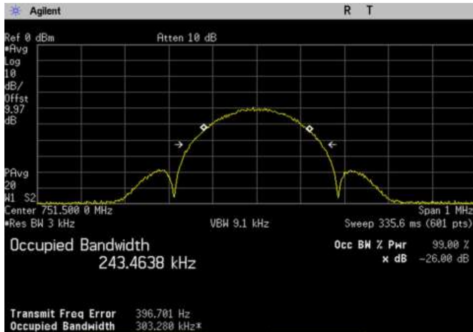
7.10 OBW-In_DL_746-757_EDGE_ 751.5MHz
