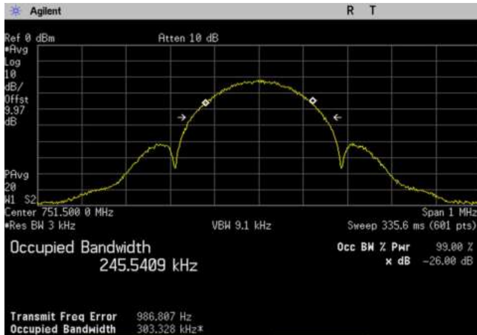
7.10 OBW-Out_DL_746-757_EDGE_ 751.5MHz
