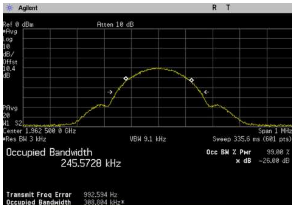
7.10 OBW-In_DL_1930-1995_GSM_1962.5MHz
