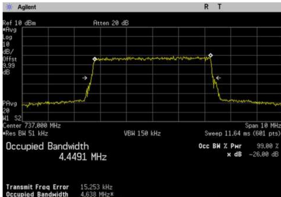
7.10 OBW-Out_DL_728-746_LTE_ 737MHz
