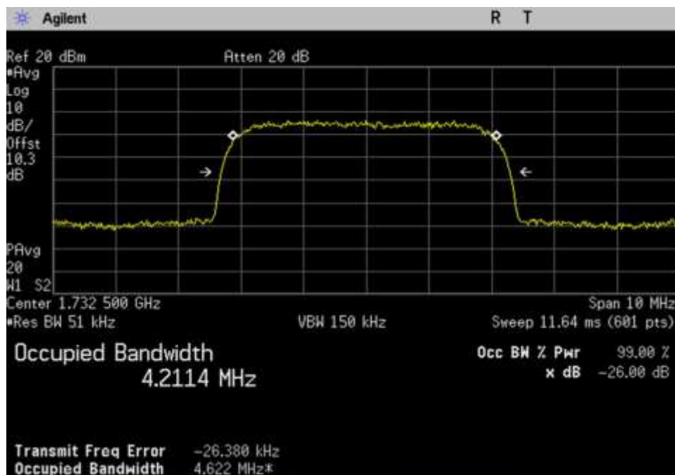
7.10 OBW-Out_UL_1710-1755_WCDMA_1732.5MHz
