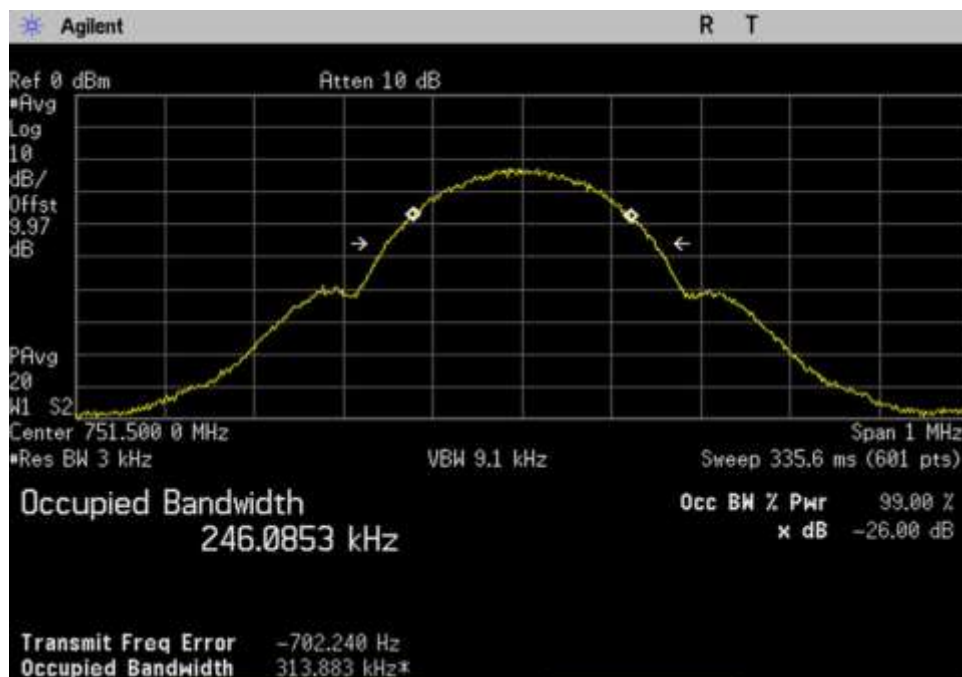
7.10 OBW-Out_DL_746-757_GSM_ 751.5MHz
