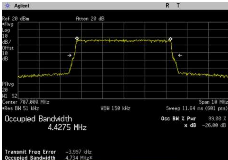
7.10 OBW-Out_UL_698-716_LTE_ 707MHz
