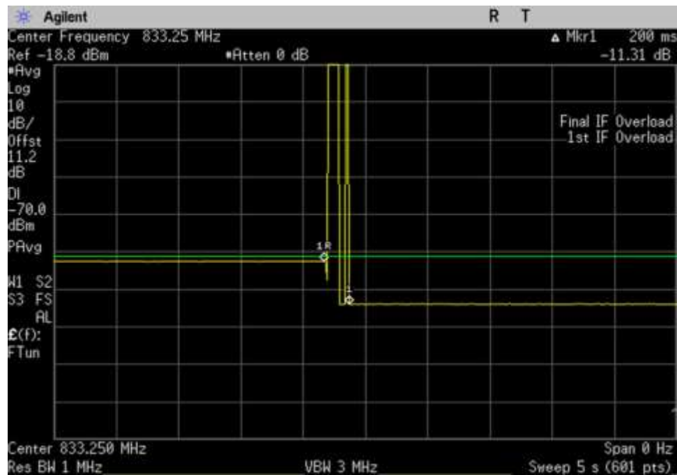
7.11.2 Osc_UL_824-849_ 833.25MHz
