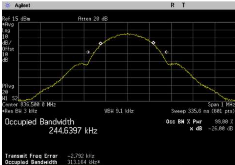
7.10 OBW-Out_UL_824-849_GSM_ 836.5MHz
