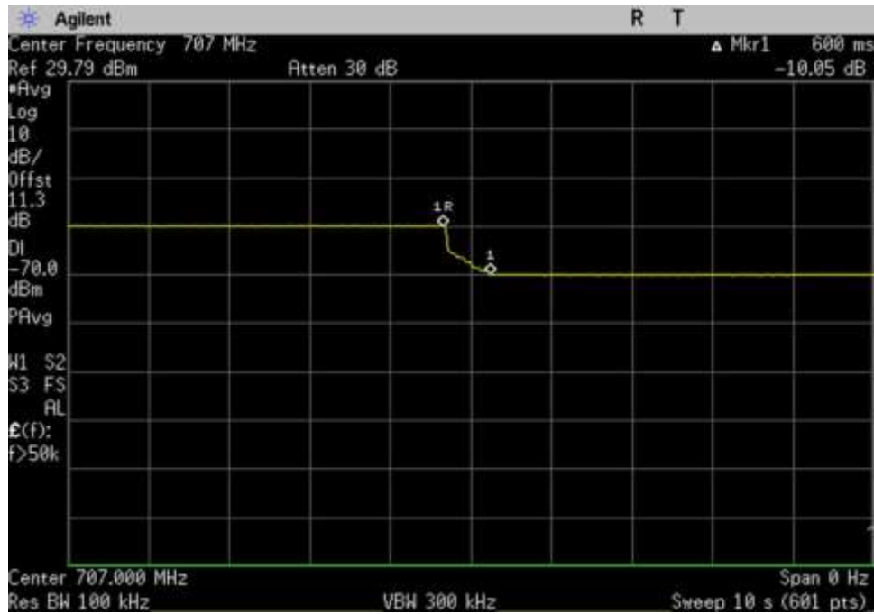
7.9 Var Gain_UL_698-716_ 707MHz_Var
