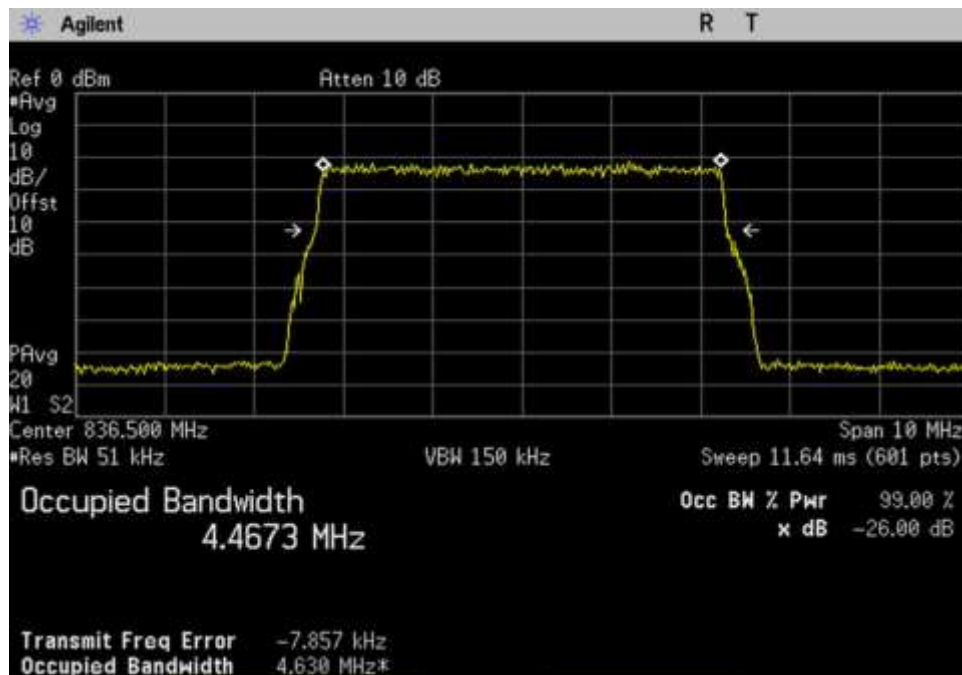
7.10 OBW-In_UL_824-849_LTE_ 836.5MHz
