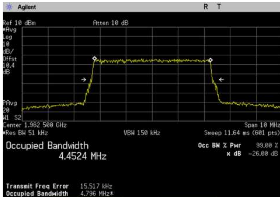
7.10 OBW-Out_DL_1930-1995_LTE_1962.5MHz
