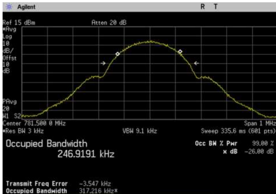
7.10 OBW-Out_UL_776-787_GSM_ 781.5MHz
