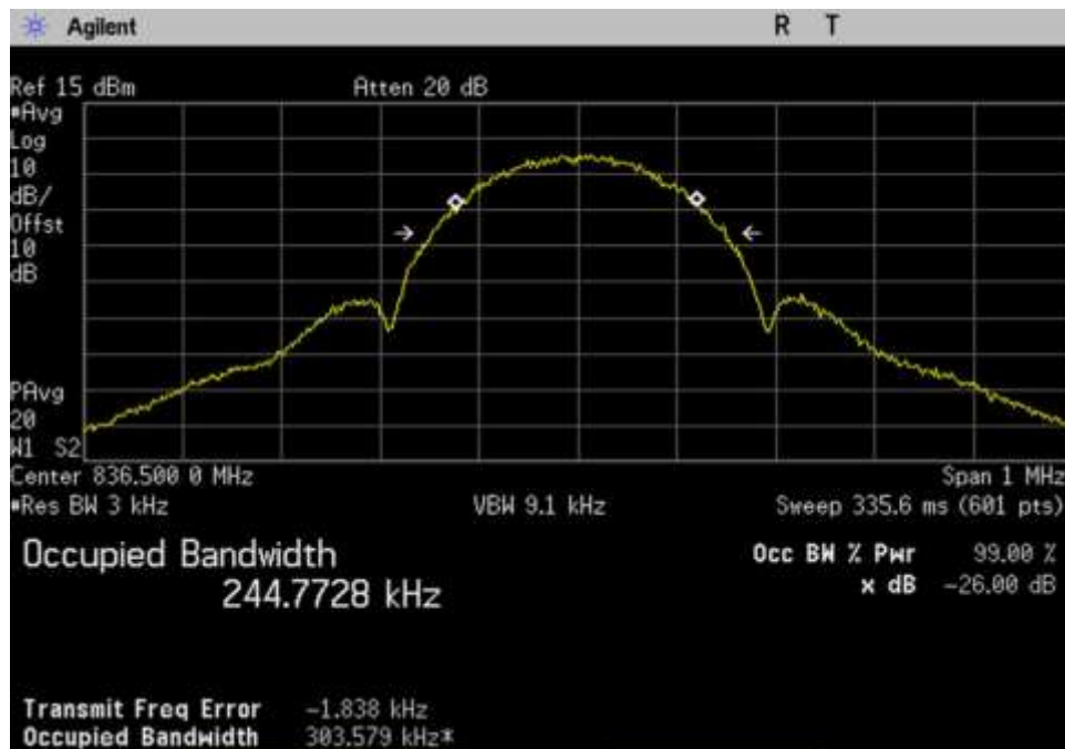
7.10 OBW-Out_UL_824-849_EDGE_ 836.5MHz
