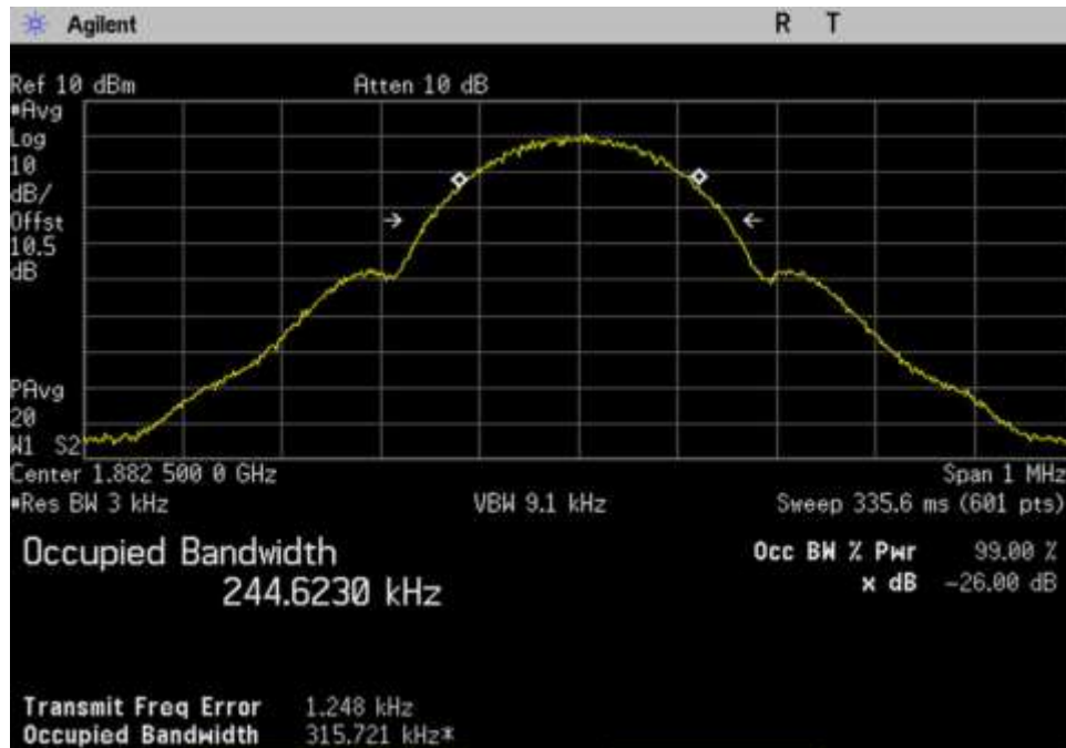
7.10 OBW-Out_UL_1850-1915_GSM_1882.5MHz
