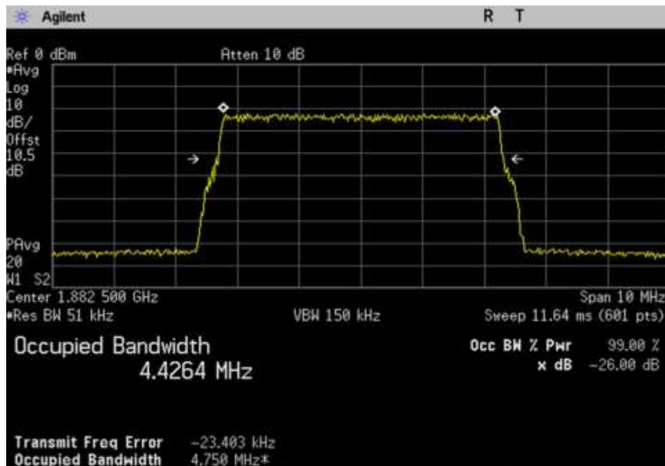
7.10 OBW-In_UL_1850-1915_LTE_ 1882.5MHz
