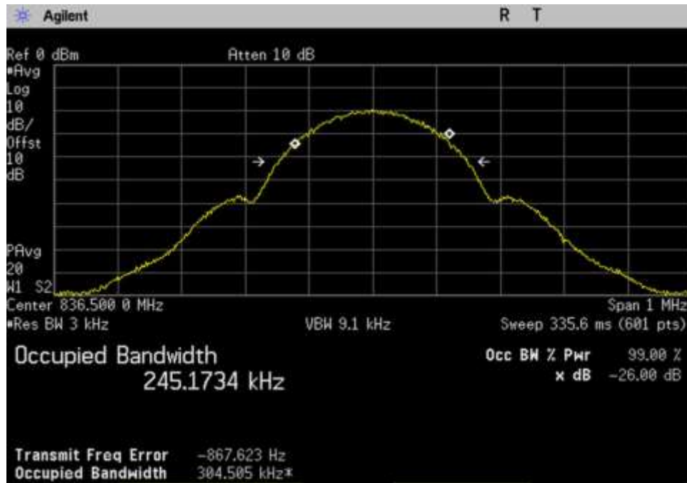
7.10 OBW-In_UL_824-849_GSM_ 836.5MHz
