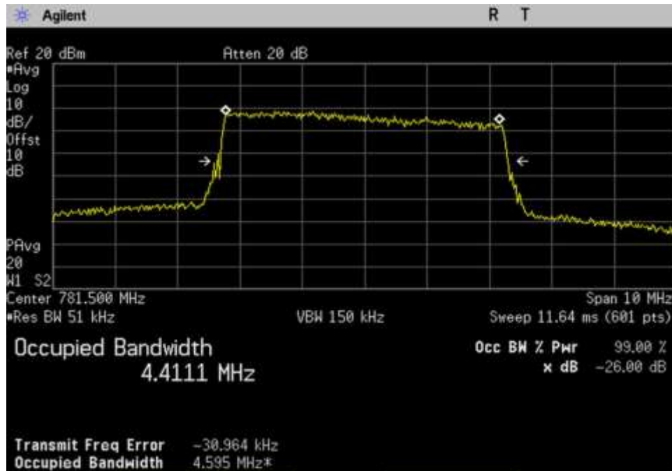
7.10 OBW-Out_UL_776-787_LTE_ 781.5MHz
