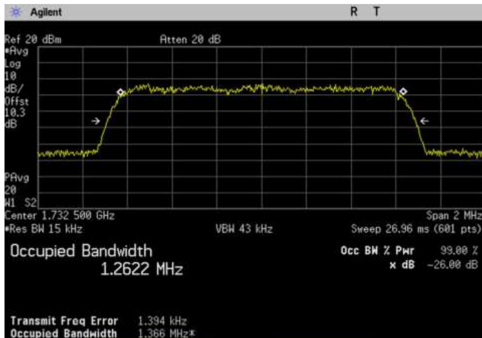
7.10 OBW-Out_UL_1710-1755_CDMA_ 1732.5MHz
