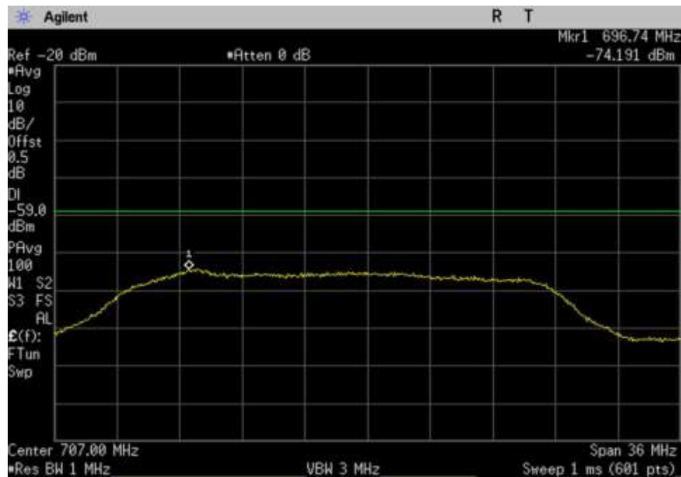
7.7 Noise_UL_698-716_ 707MHz
