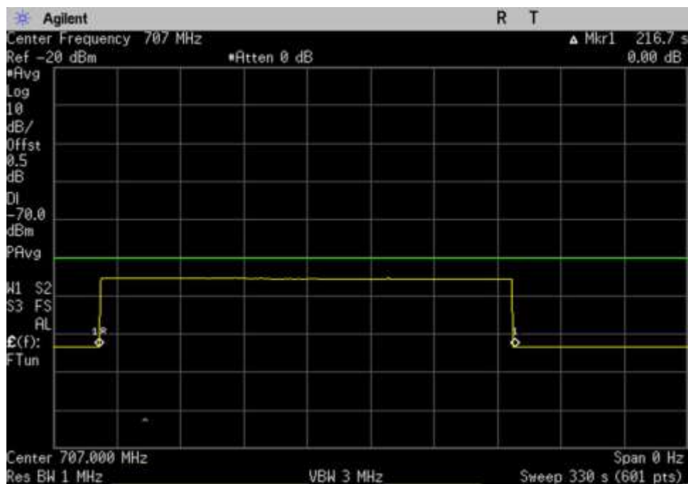
7.8 Inact_UL_698-716_ 707MHz
