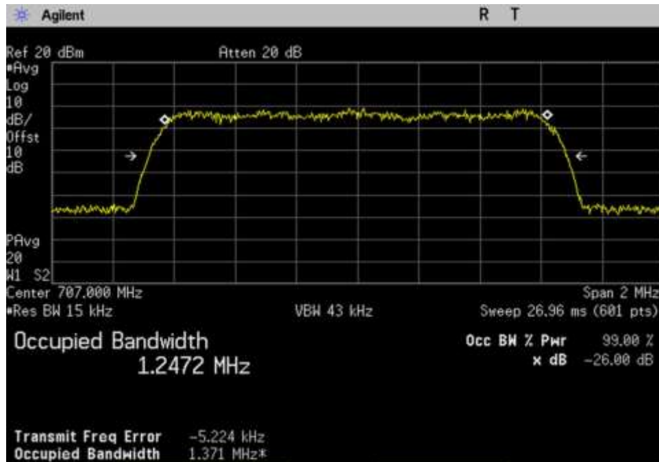
7.10 OBW-Out_UL_698-716_CDMA_707MHz
