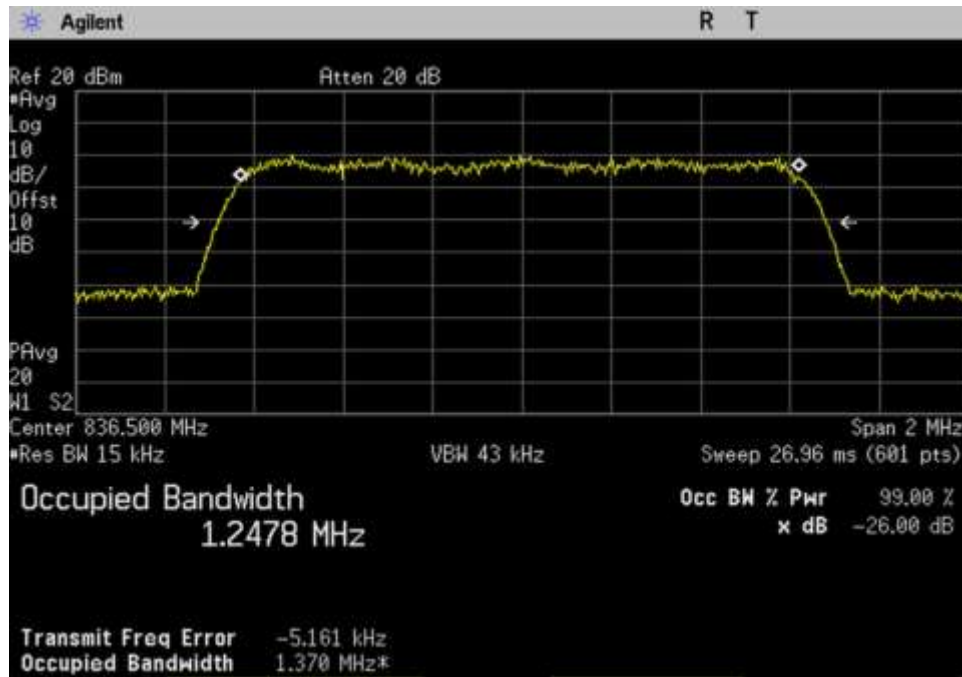
7.10 OBW-Out_UL_824-849_CDMA_ 836.5MHz
