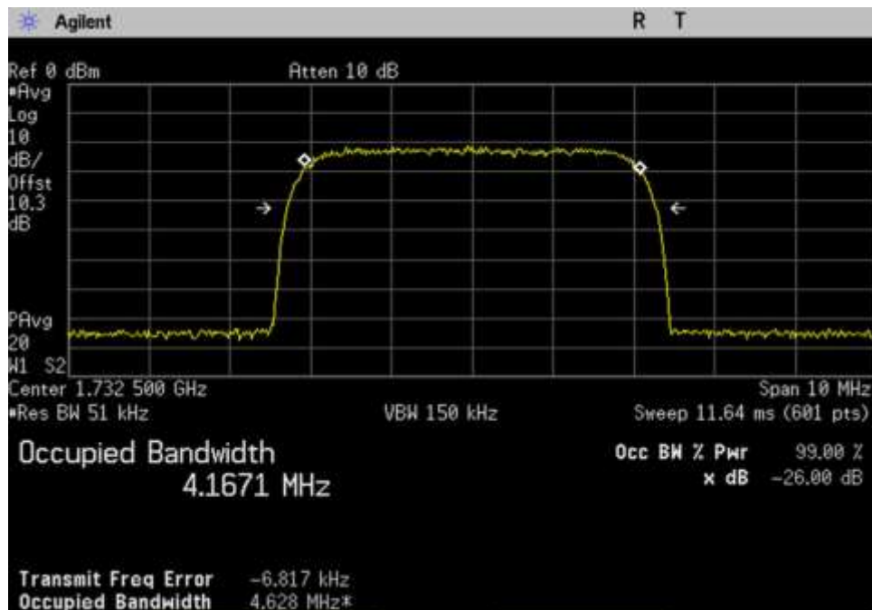
7.10 OBW-In_UL_1710-1755_WCDMA_ 1732.5MHz
