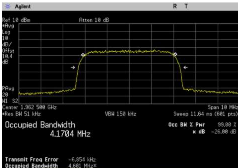
7.10 OBW-Out_DL_1930-1995_WCDMA_1962.5MHz
