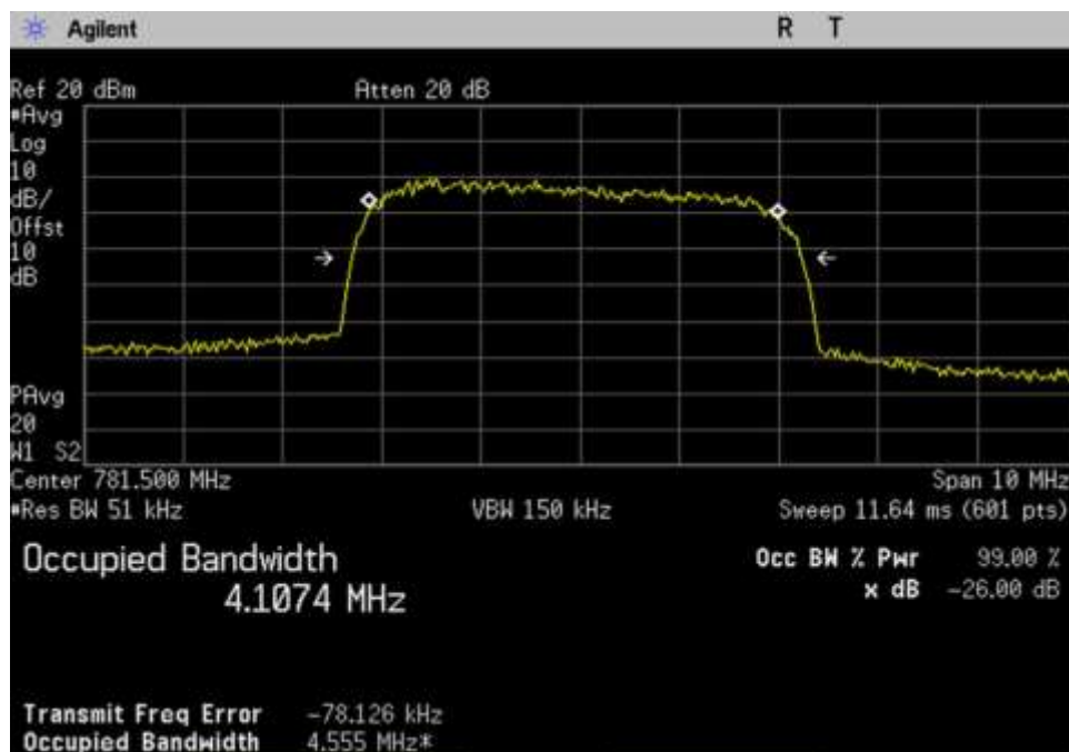
7.10 OBW-Out_UL_776-787_WCDMA_ 781.5MHz
