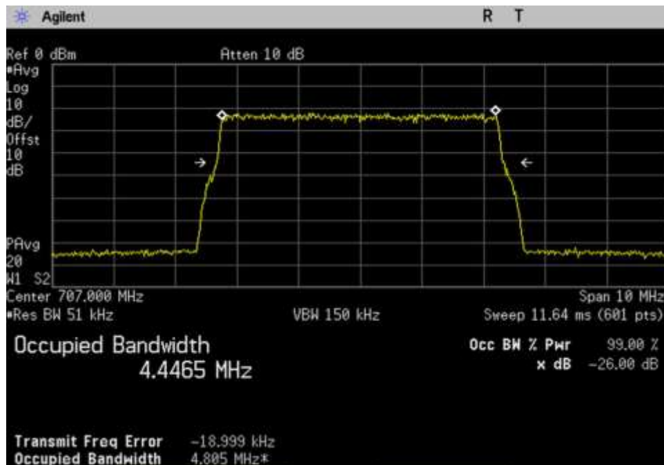
7.10 OBW-In_UL_698-716_LTE_707MHz
