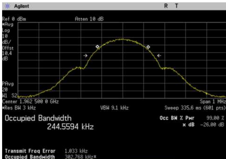
7.10 OBW-Out_DL_1930-1995_GSM_ 1962.5MHz
