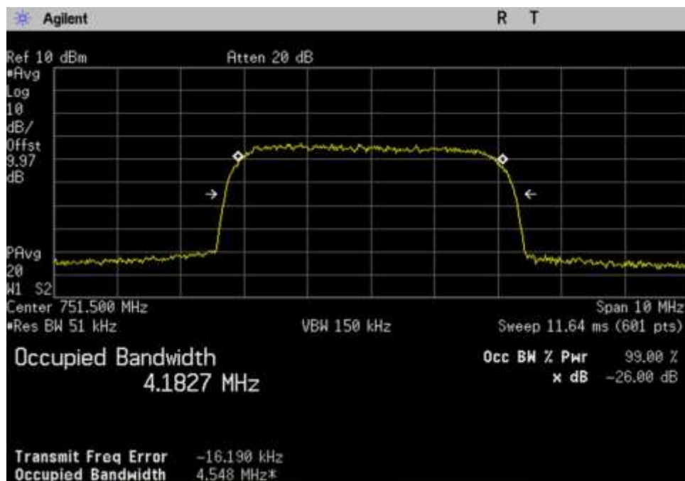
7.10 OBW-Out_DL_746-757_WCDMA_751.5MHz
