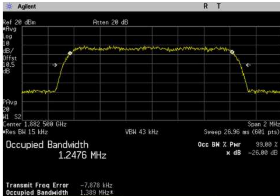
7.10 OBW-Out_UL_1850-1915_CDMA_ 1882.5MHz
