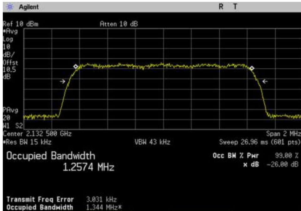
7.10 OBW-Out_DL_2110-2155_CDMA_ 2132.5MHz
