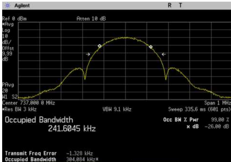
7.10 OBW-Out_DL_728-746_EDGE_737MHz
