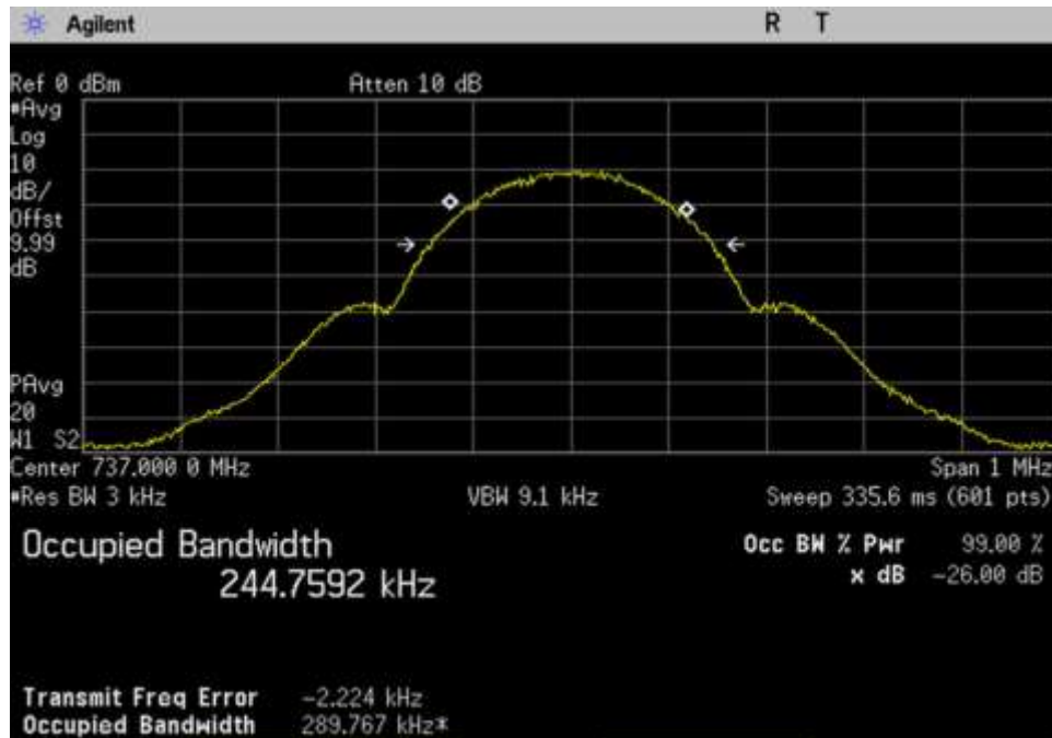
7.10 OBW-Out_DL_728-746_GSM_ 737MHz
