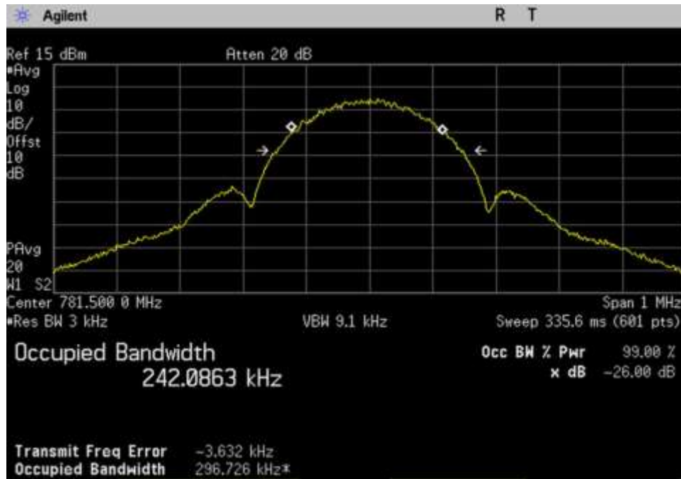
7.10 OBW-Out_UL_776-787_EDGE_ 781.5MHz
