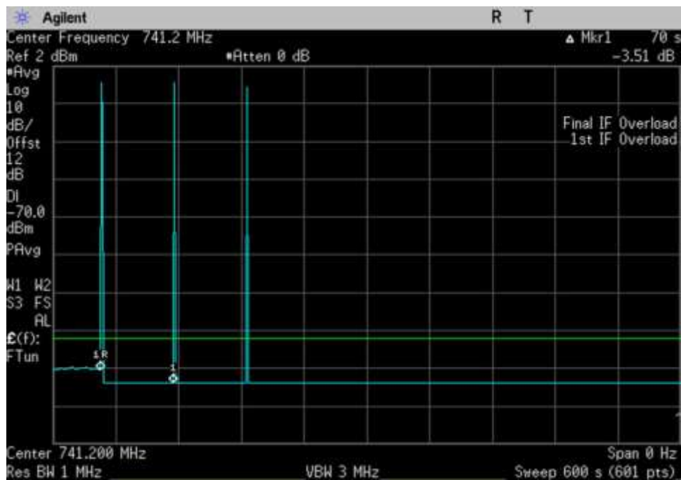
7.11.2 Osc_DL_728-746_600sec_741.2MHz
