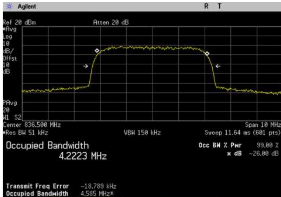
7.10 OBW-Out_UL_824-849_WCDMA_ 836.5MHz
