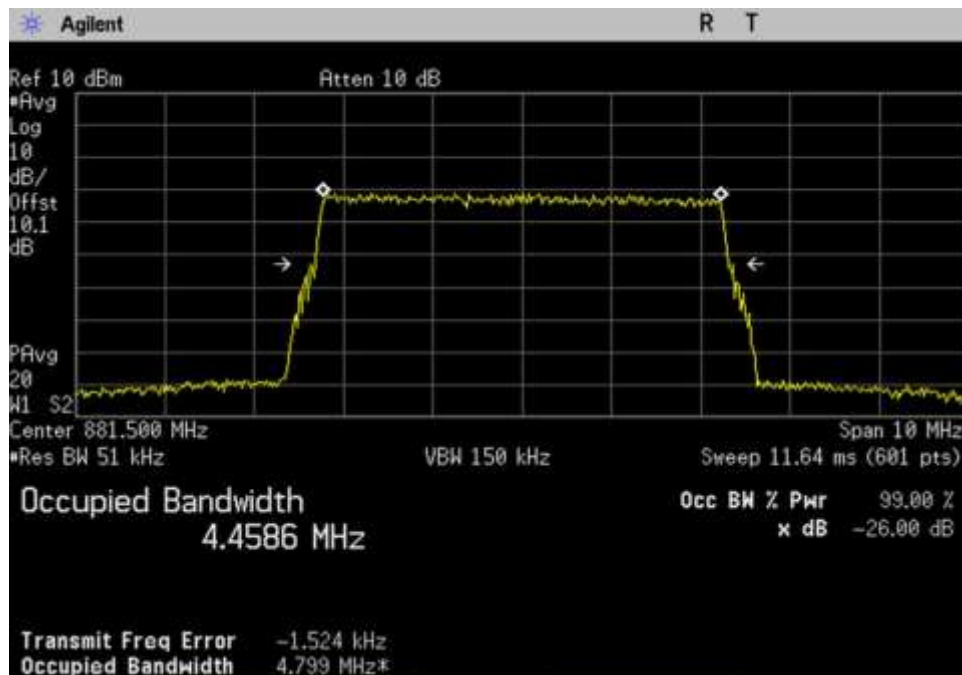
7.10 OBW-Out_DL_869-894_LTE_ 881.5MHz
