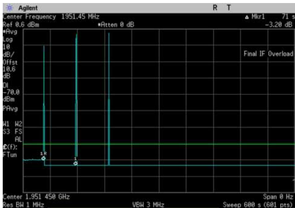
7.11.2 Osc_DL_1930-1995_600sec_ 1951.45MHz
