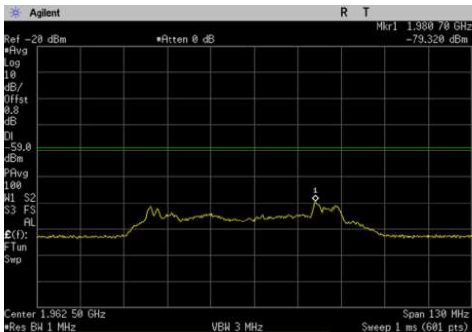
7.7 Noise_DL_1930-1995_ 1962.5MHz
