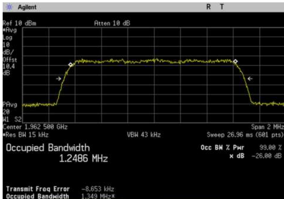
7.10 OBW-Out_DL_1930-1995_CDMA_ 1962.5MHz
