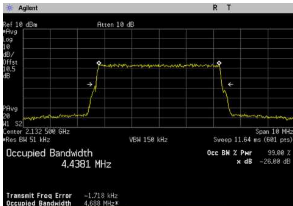
7.10 OBW-Out_DL_2110-2155_LTE_ 2132.5MHz
