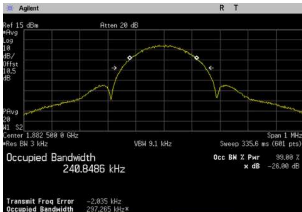
7.10 OBW-Out_UL_1850-1915_EDGE_ 1882.5MHz
