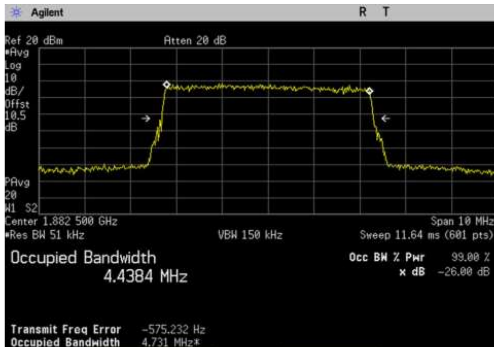
7.10 OBW-Out_UL_1850-1915_LTE_1882.5MHz
