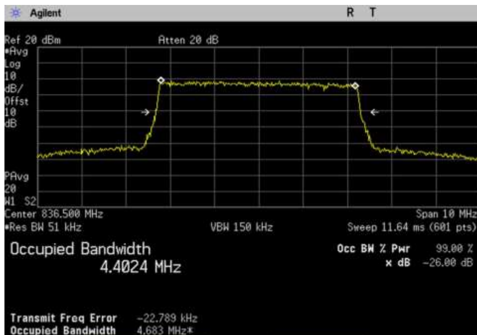
7.10 OBW-Out_UL_824-849_LTE_ 836.5MHz
