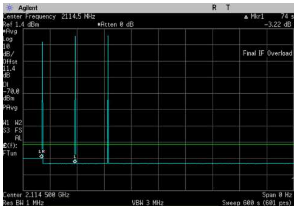
7.11.2 Osc_DL_2110-2155_600sec_ 2114.5MHz
