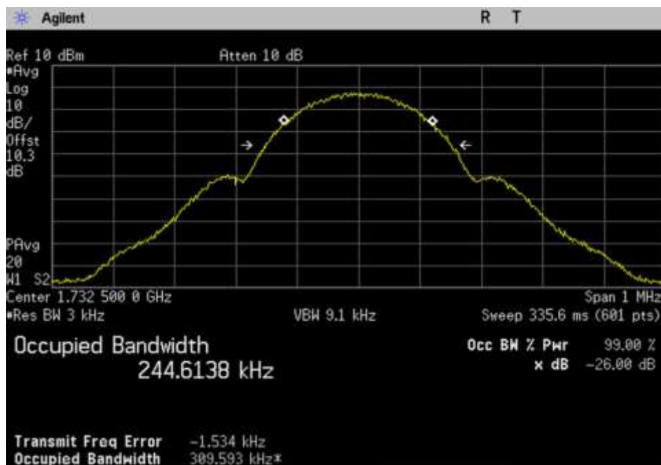
7.10 OBW-Out_UL_1710-1755_GSM_ 1732.5MHz
