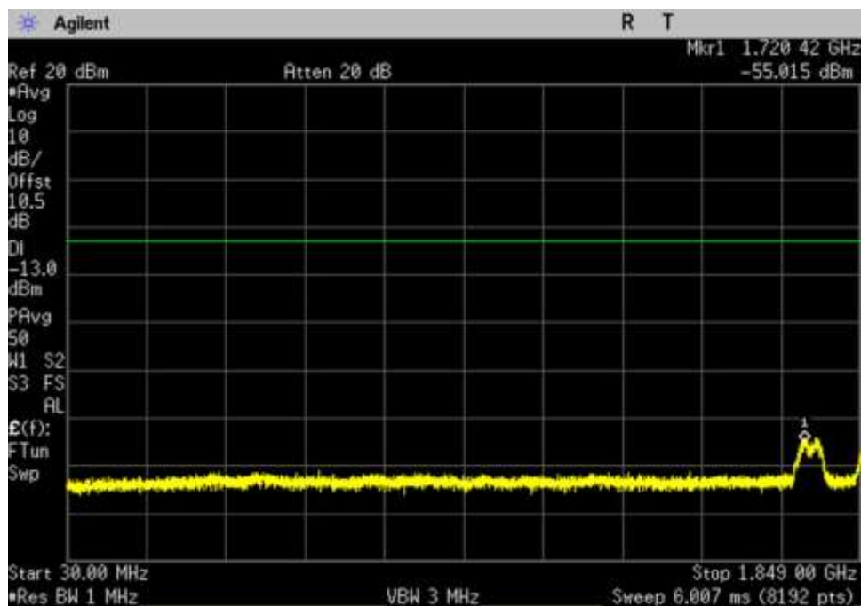
7.6 CSE_UL_1850-1915_ 30- 1849MHz
