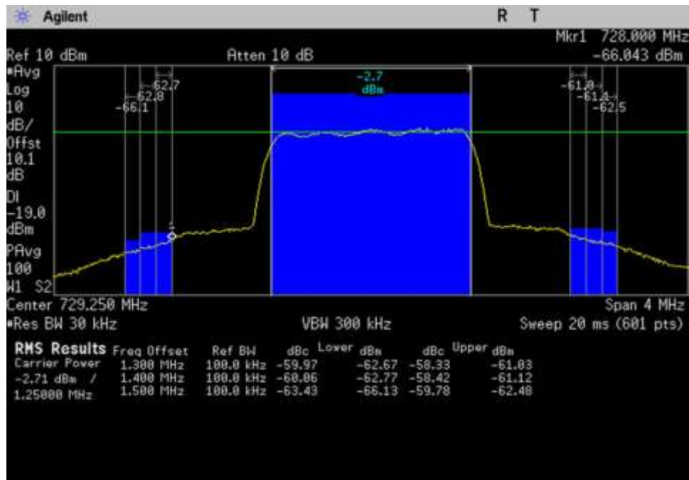
7.5 OBE_DL_728-746_CDMA_ 727.25- 731.25MHz
