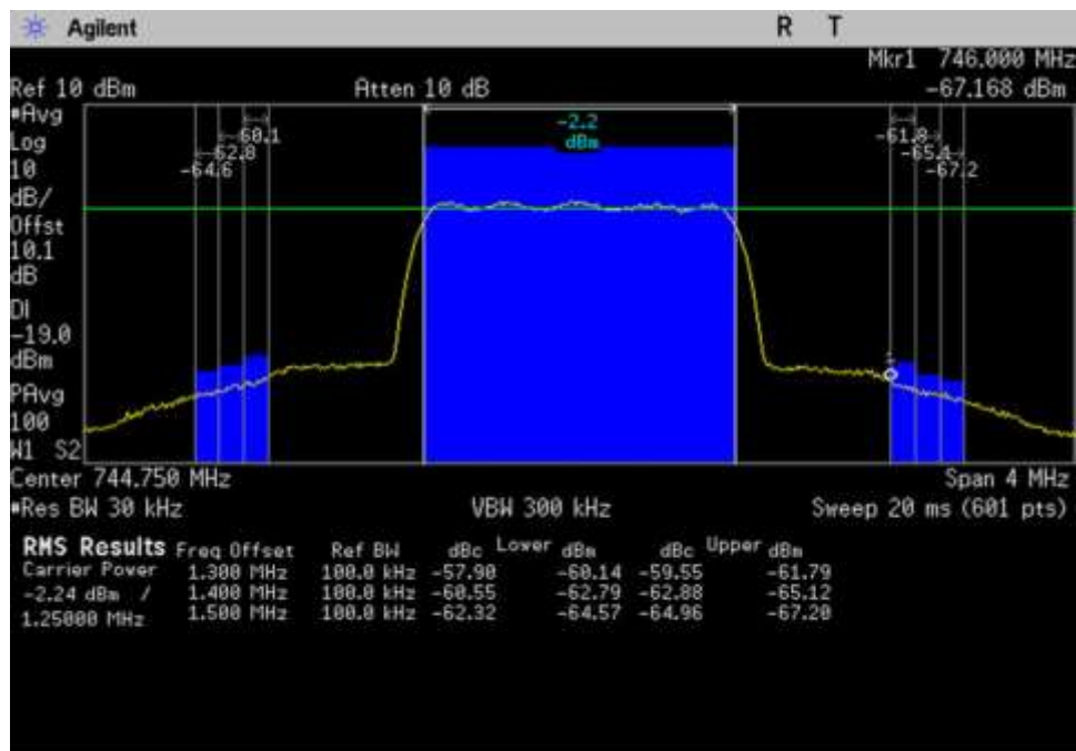
7.5 OBE_DL_728-746_CDMA_ 742.75- 746.75MHz
