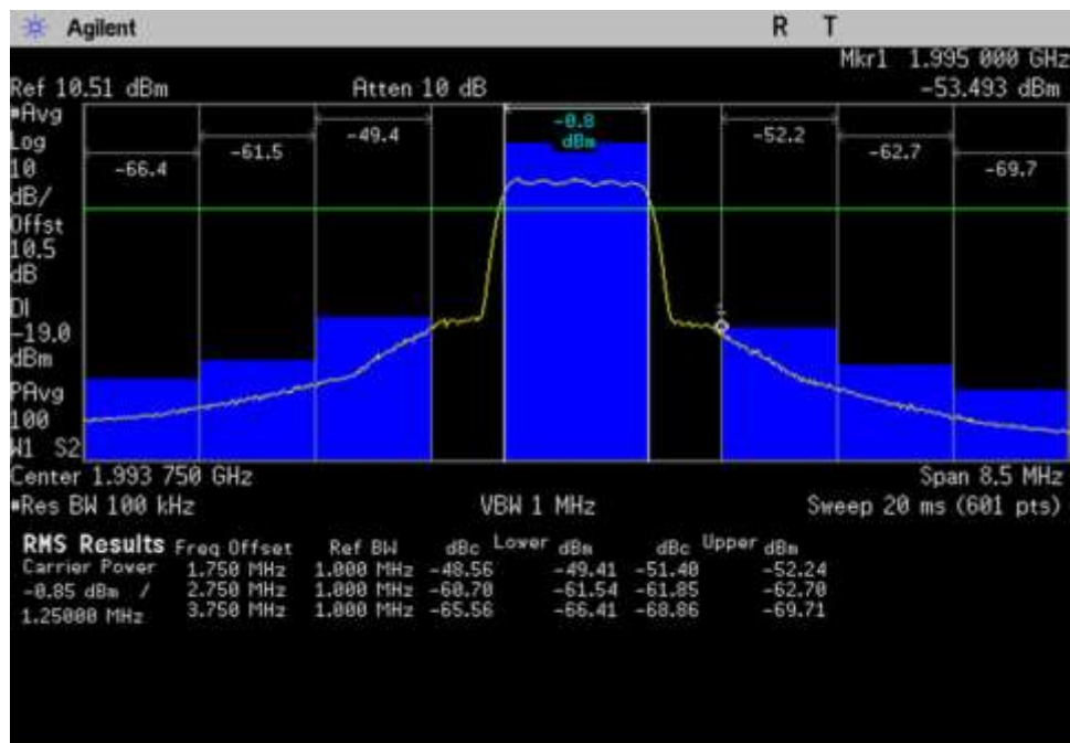
7.5 OBE_DL_1930-1995_CDMA_1989.5- 1998MHz
