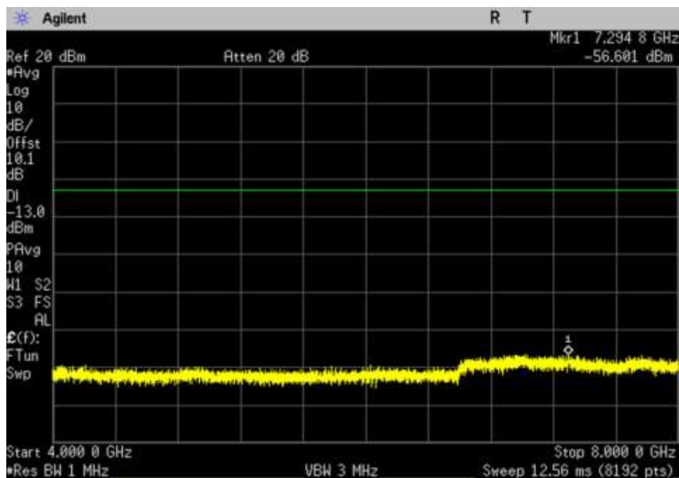
7.6 CSE_DL_746-757_ 4000- 8000MHz
