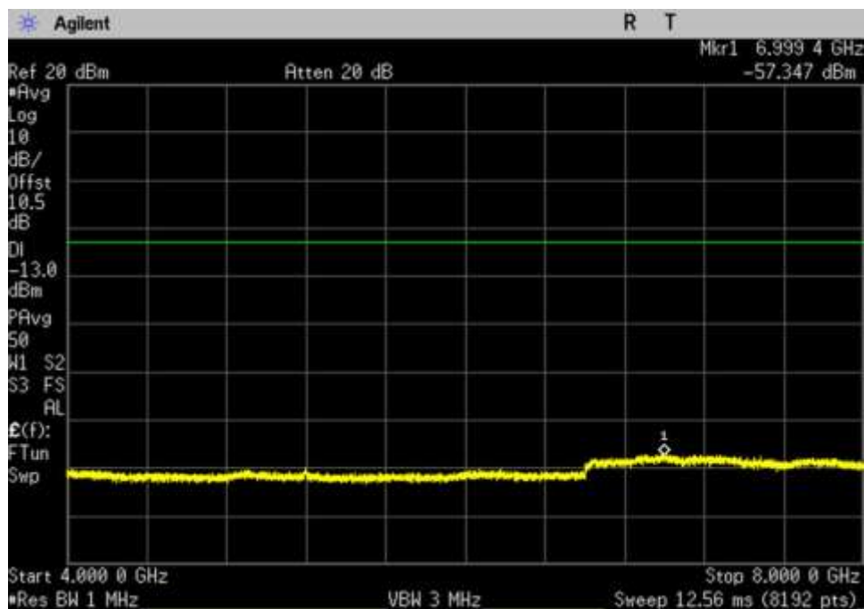
7.6 CSE_UL_1710-1755_ 4000- 8000MHz
