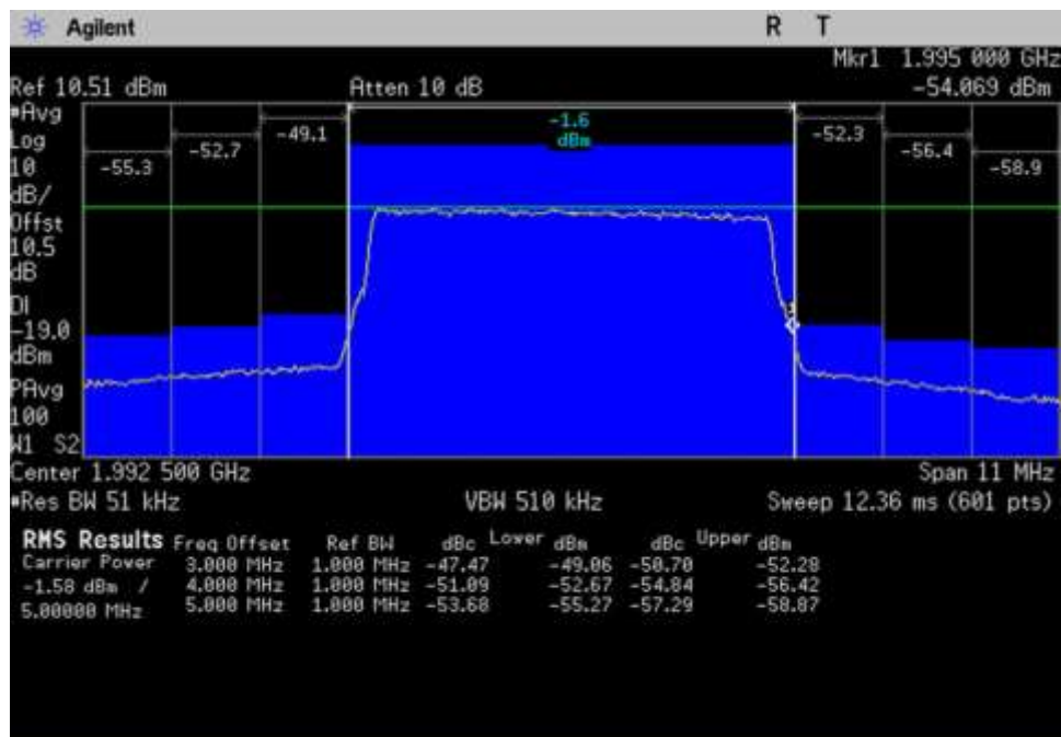
7.5 OBE_DL_1930-1995_LTE_1987-1998MHz
