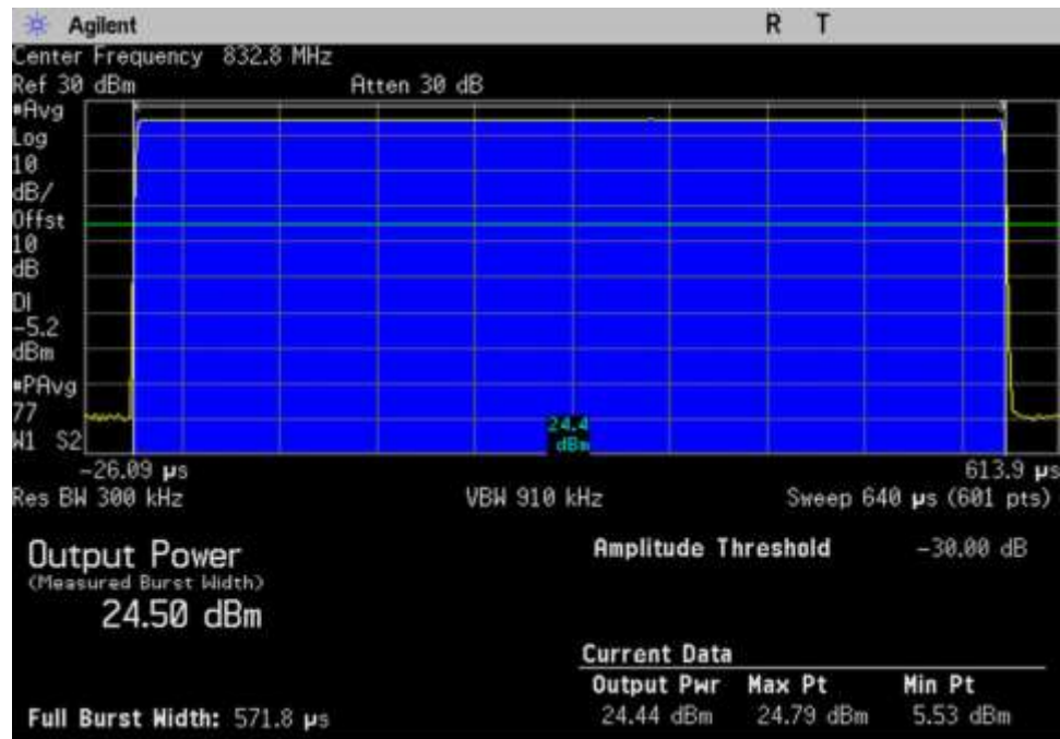
7.2-7.3 Power Gain_UL_824-849_GSM_ 832.8MHz
