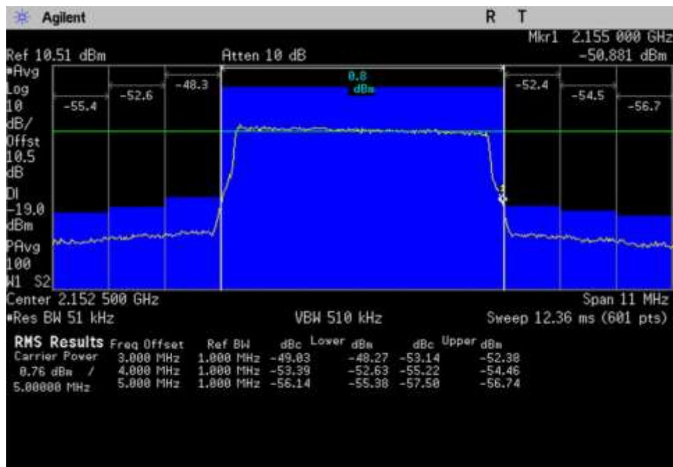
7.5 OBE_DL_2110-2155_LTE_2147-2158MHz
