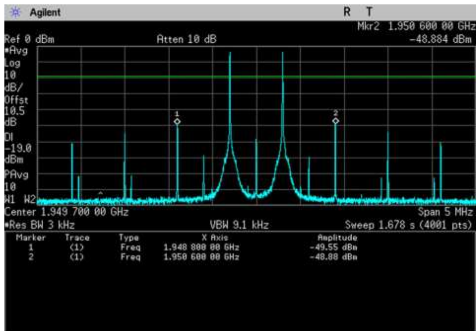
7.4 Intermod_DL_1930-1995_ 1949.7MHz
