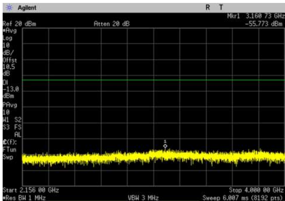
7.6 CSE_DL_2110-2155_2156-4000MHz
