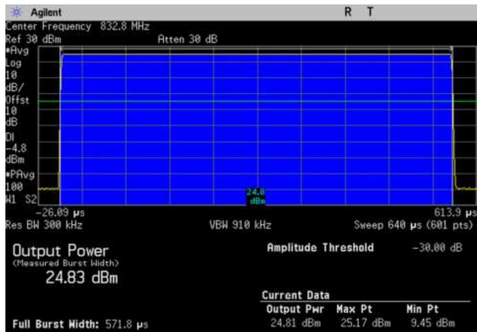
7.2-7.3 Power Gain_UL_824-849_GSM_Max_ 832.8MHz
