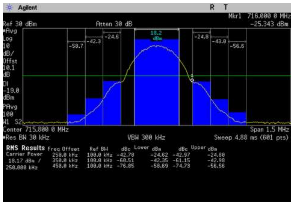
7.5 OBE_UL_698-716_GSM_ 715.05- 716.55MHz
