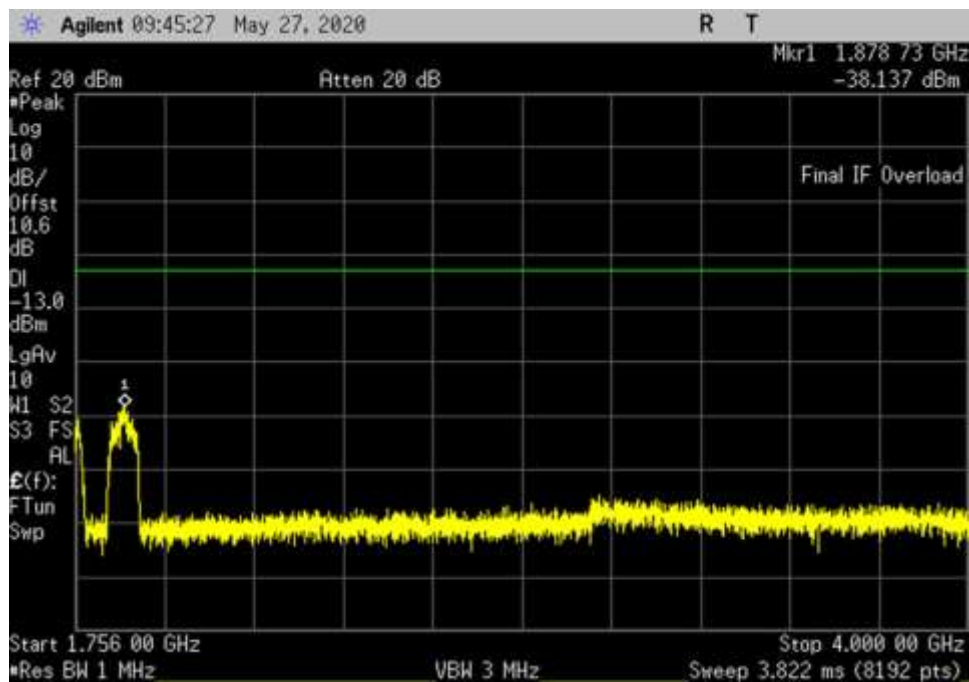
UL_1710-1755_ 1756- 4000MHz
