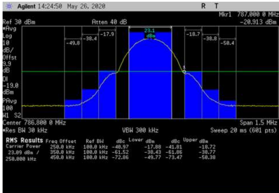
UL_776-787_GSM_786.05- 787.55MHz
