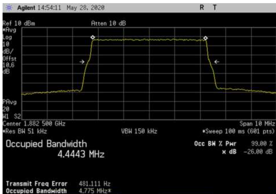
UL_1850-1915_LTE_ 1882.5MHz
