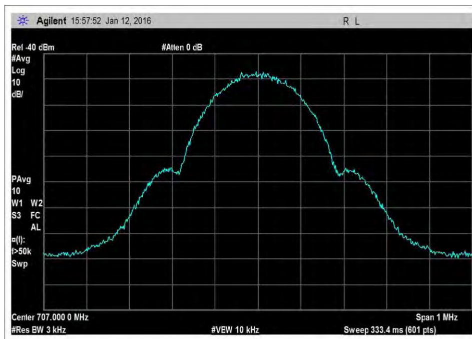
7.10_OBW_UL_698-716MHz_GSM
