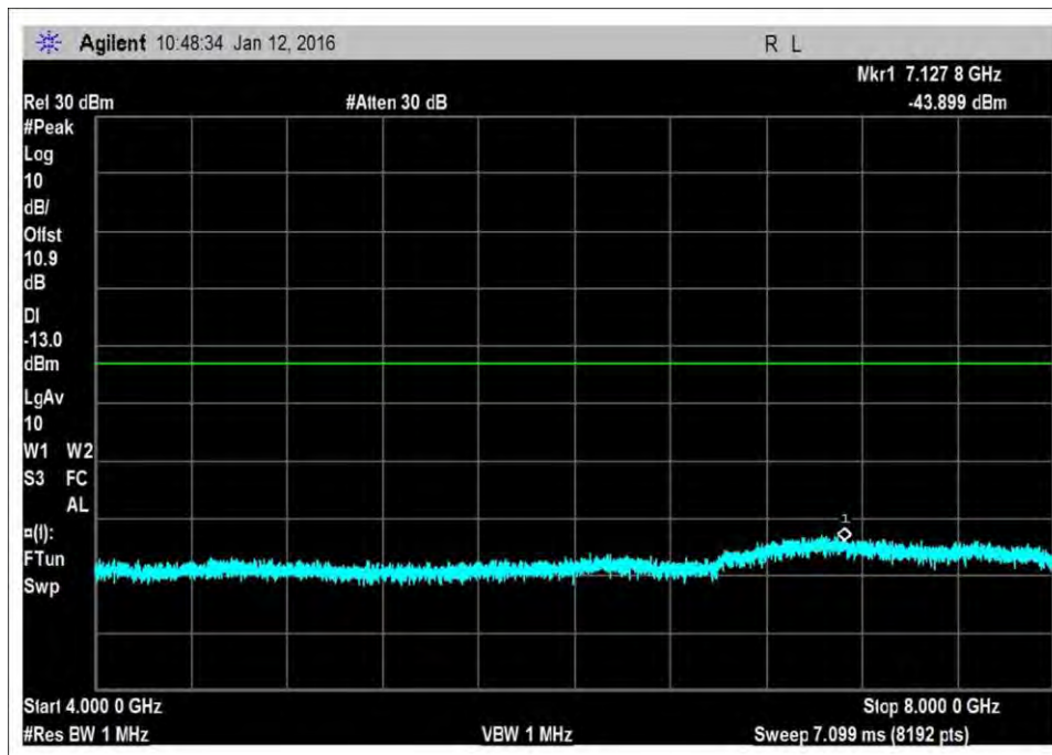
UL_1710-1755R2
