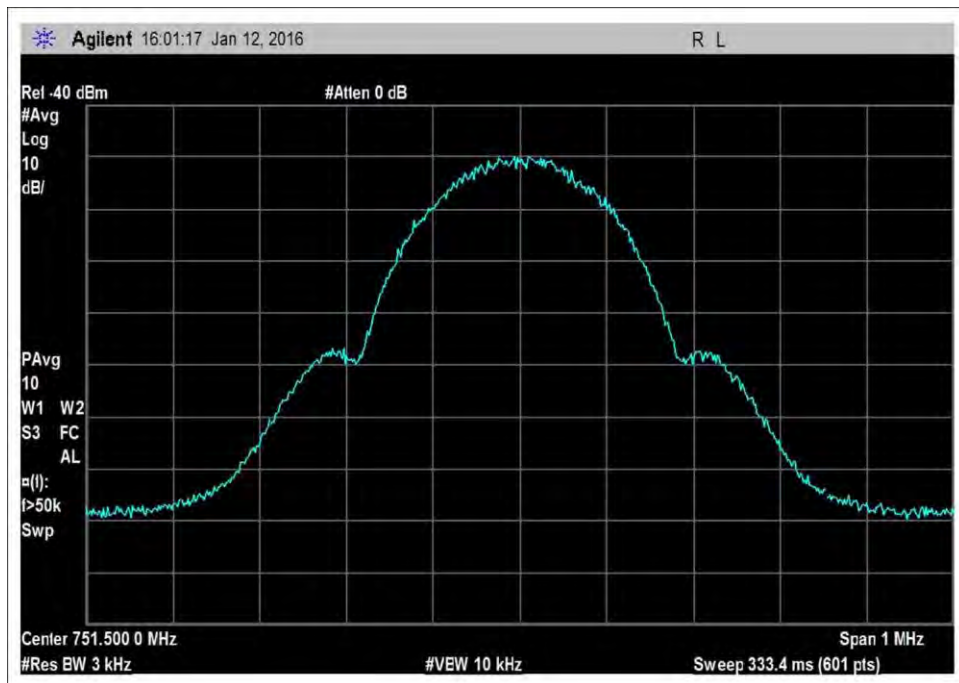
7.10_OBW_DL_746-757MHz_GSM
