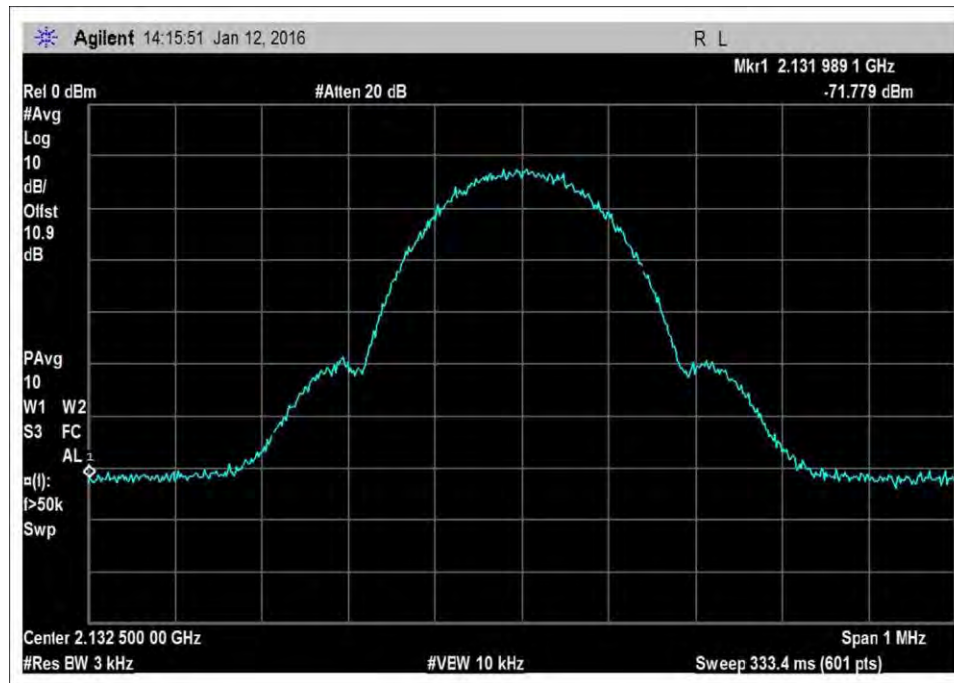
7.10_OBW_DL_2110-2155MHz_GSM
