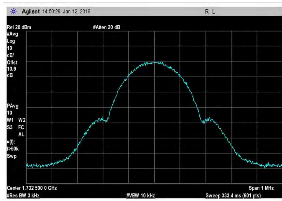
7.10_OBW_UL_1710-1755MHz_GSM
