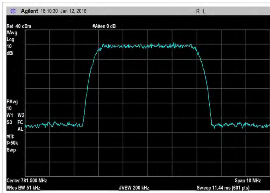
7.10_OBW_UL_776-787MHz_WCDMA
