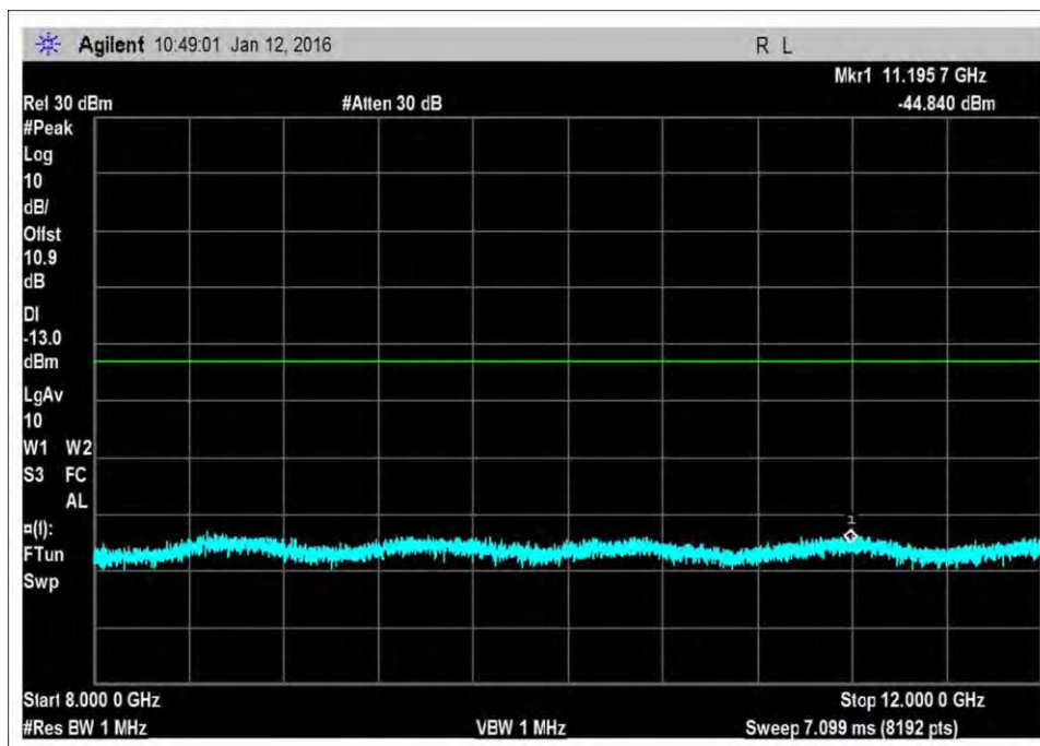
UL_1710-1755R3
