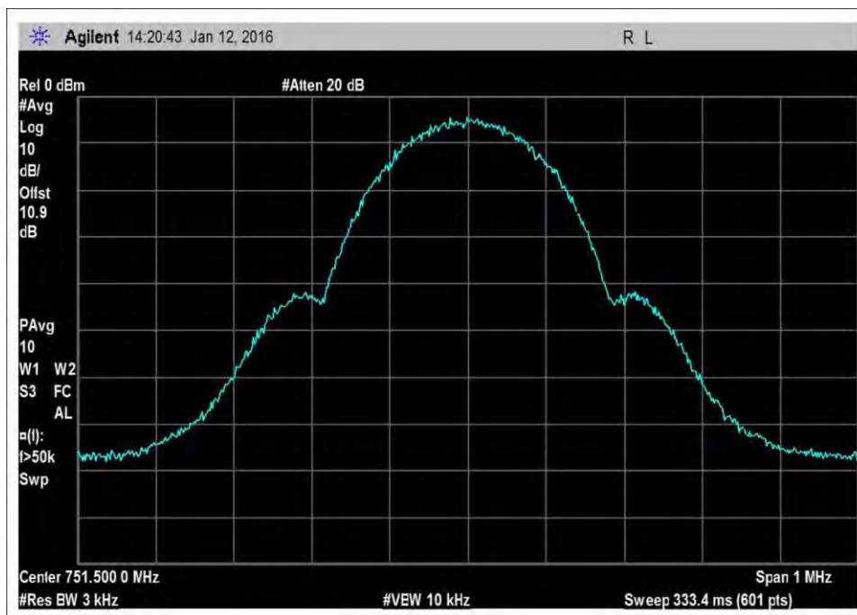
7.10_OBW_DL_746-757MHz_GSM
