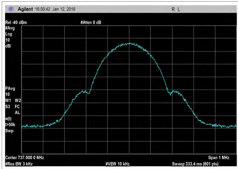
7.10_OBW_DL_728-746MHz_GSM
