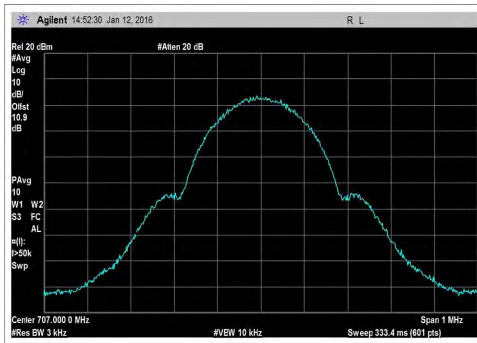
7.10_OBW_UL_698-716MHz_GSM
