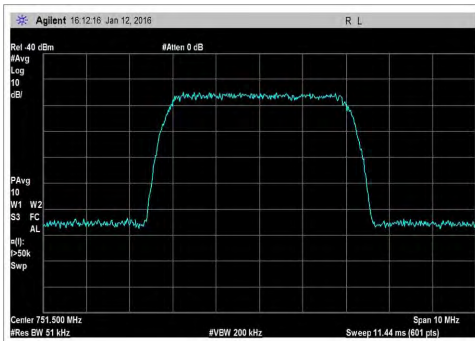
7.10_OBW_DL_746-757MHz_WCDMA
