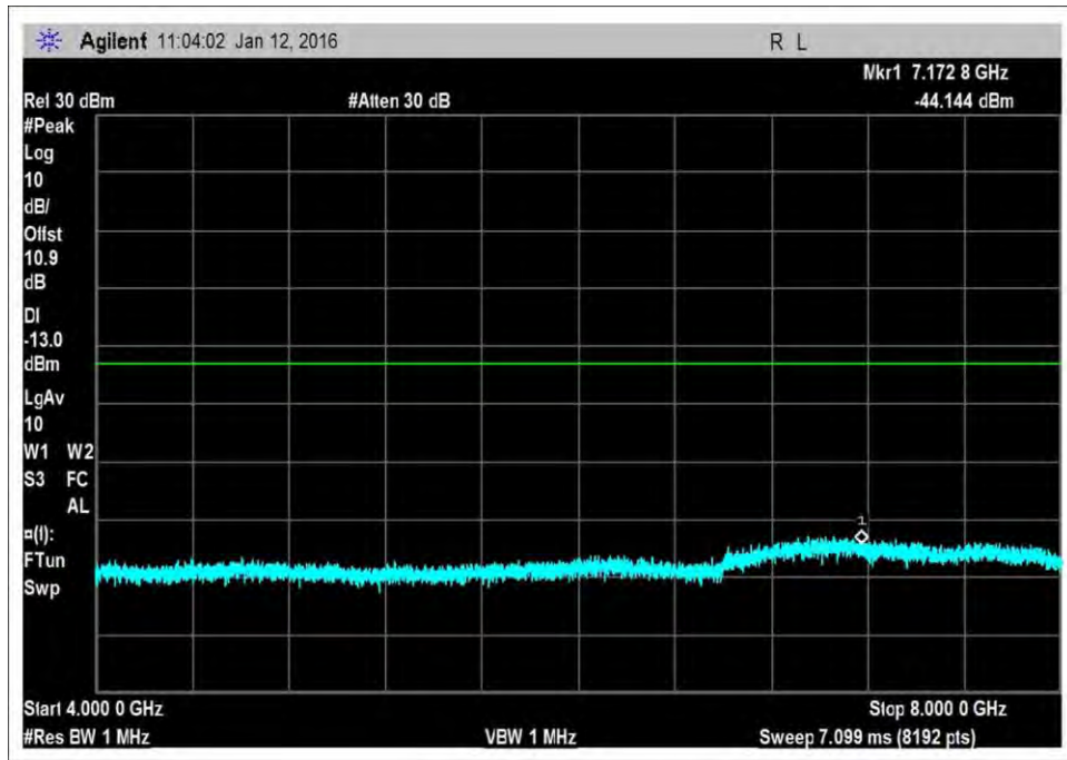
UL_698-716R2
