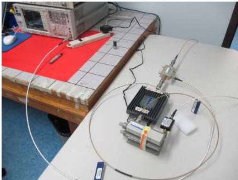
7.7.2 Test Setup
