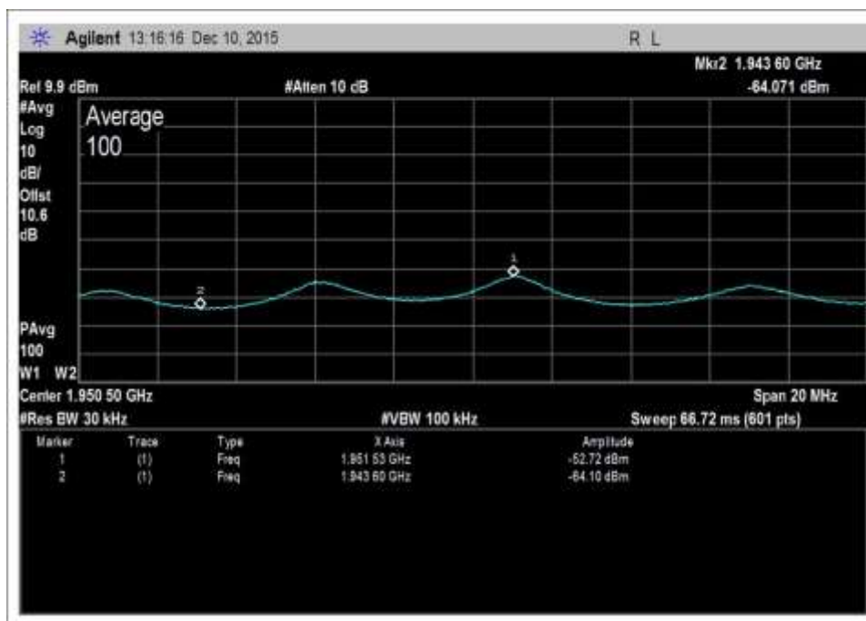
DL-1930-1995-AWGNR+2
