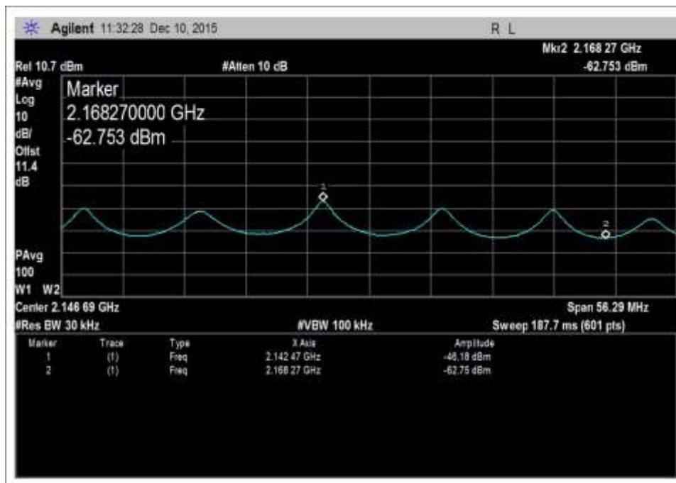
DL-2110-2155-AWGNL-2
