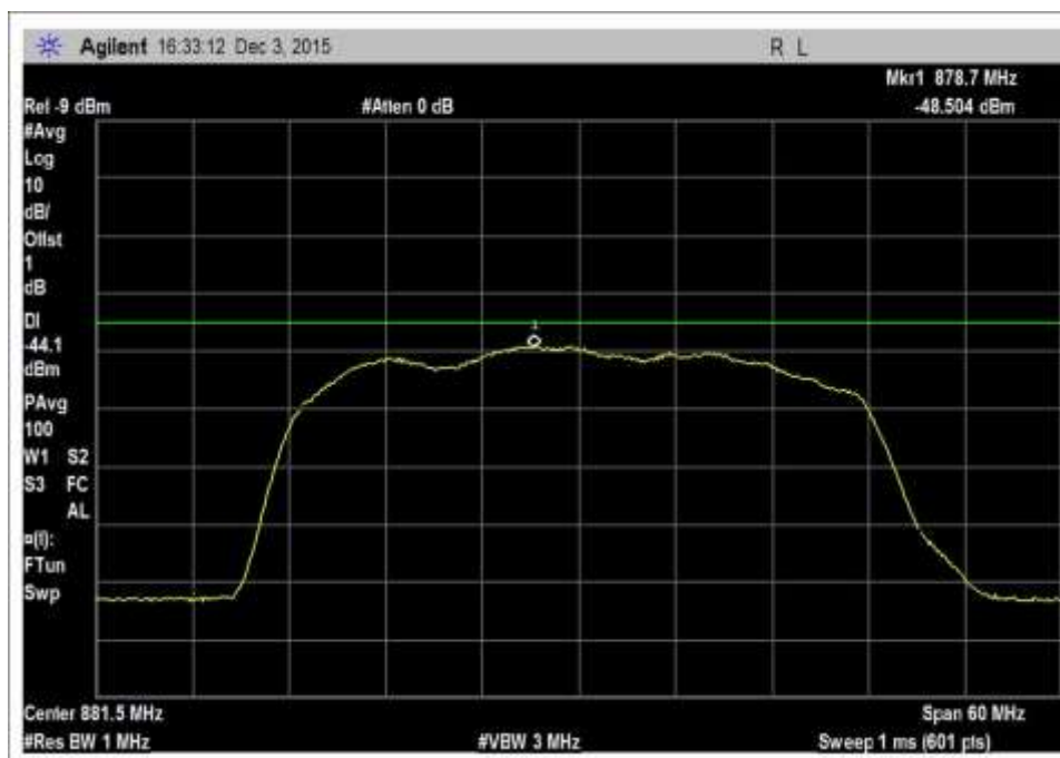
7.7_Noise_DL_869-894MHz-Zoom
