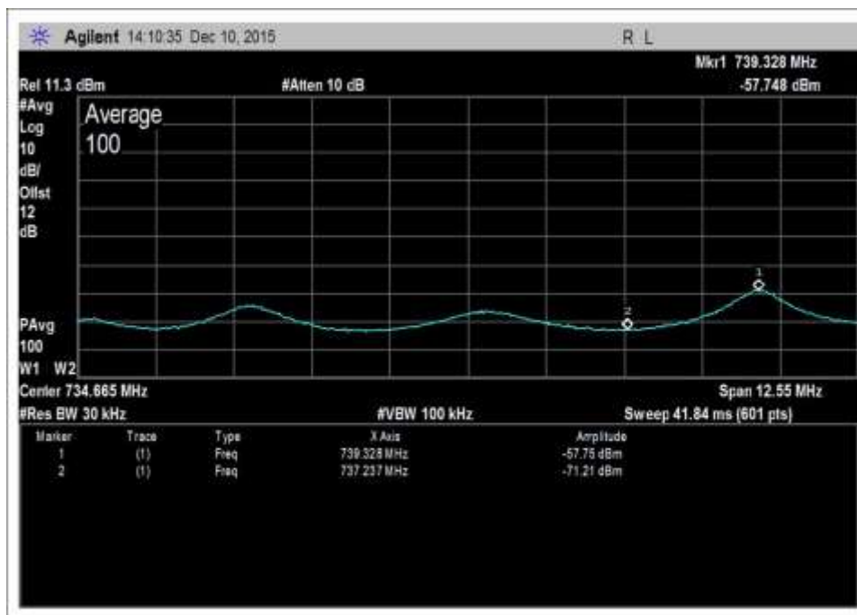
DL-728-746-AWGNR+2
