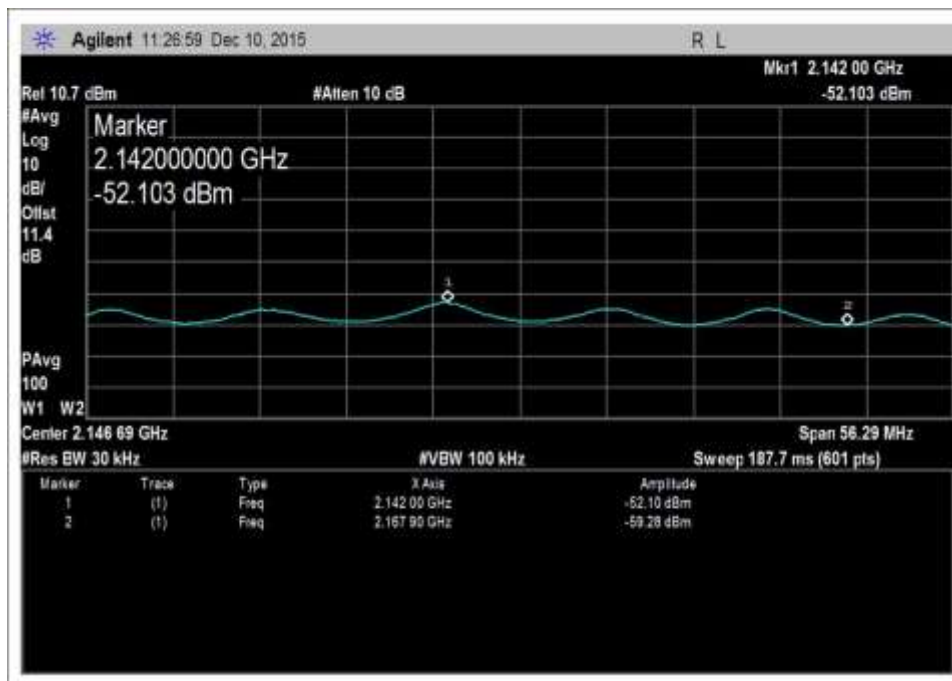
DL-2110-2155-AWGNL+5
