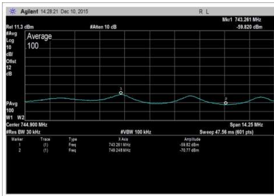
DL-746-757-AWG NR+3
