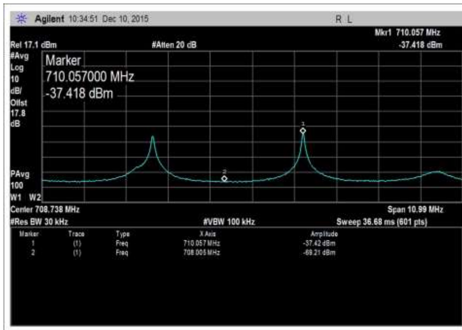
UL-698-716-AWGNL-1
