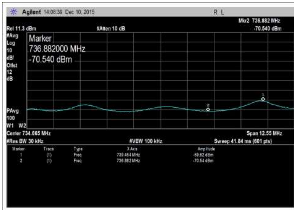
DL-728-746-AWGNR+4
