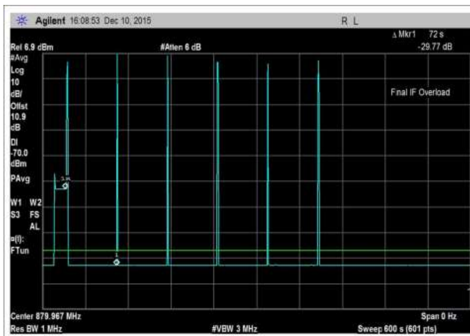
7.11_osc_DL-869-894MHz-600
