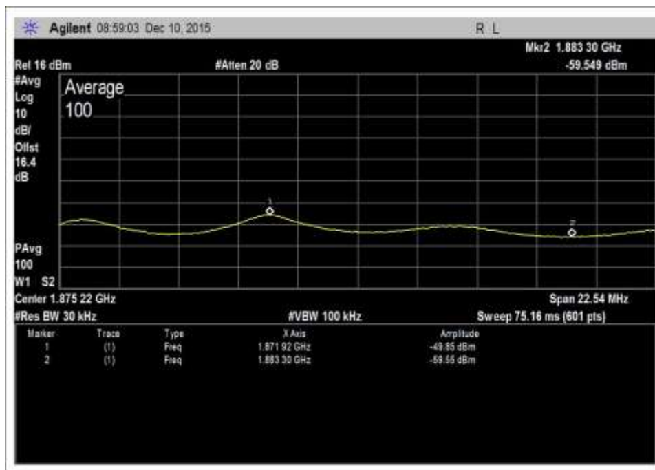
UL-1850-1915-AWGNR+4
