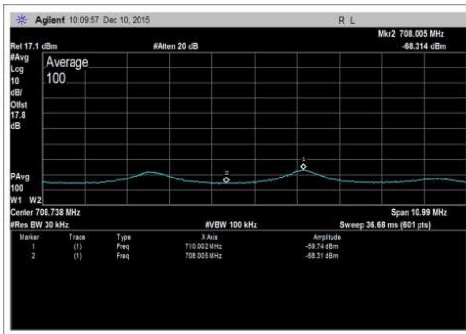
UL-698-716-AWGNL+4
