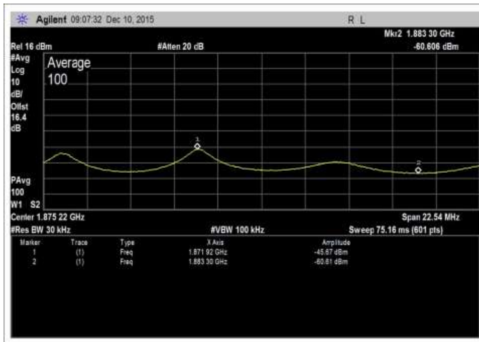
UL-1850-1915-AWGNR+0
