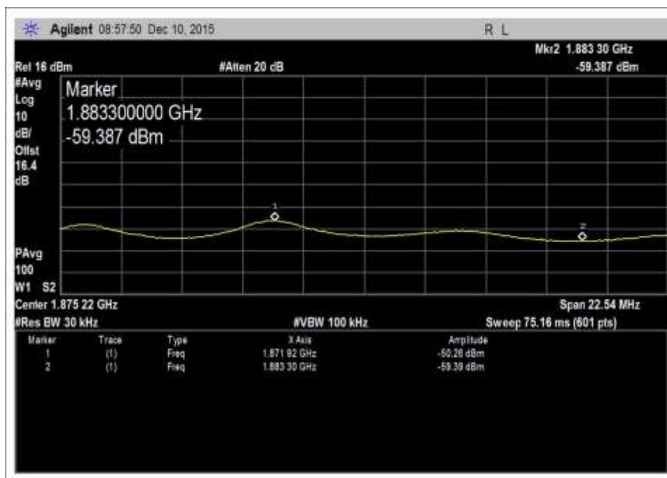
UL-1850-1915-AWGNR+5
