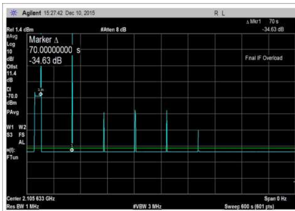
7.11_osc_DL-2110-2155MHz-600sec
