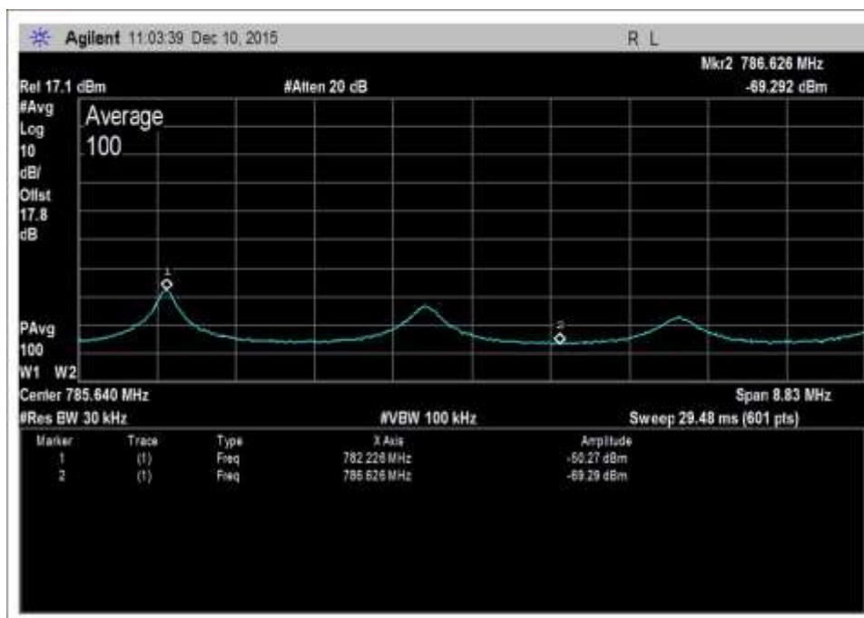
UL-776-787-AWGNL+0
