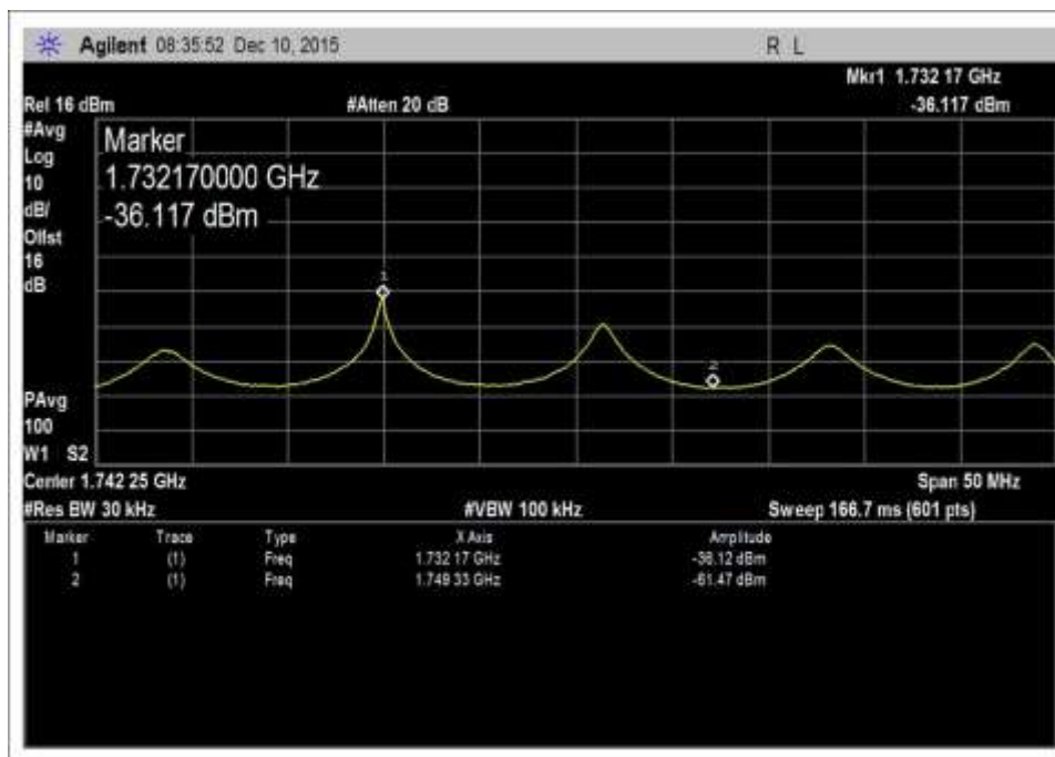
UL-1710-1755-AWGNL+0
