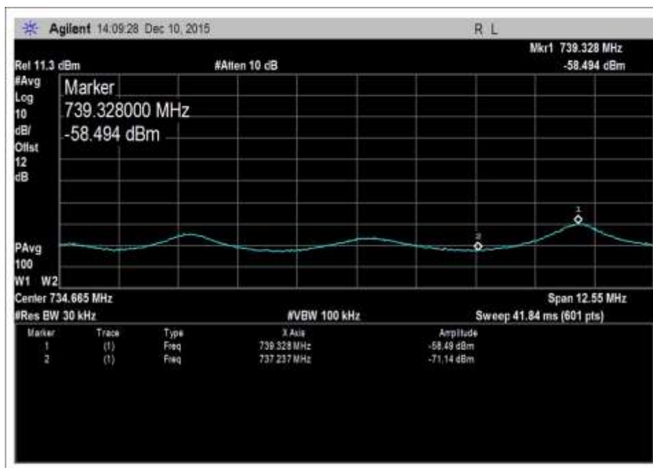
DL-728-746-AWGNR+3
