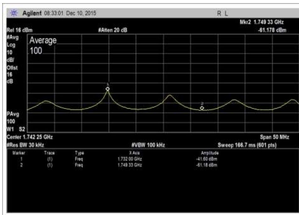
UL-1710-1755-AWGNL+1
