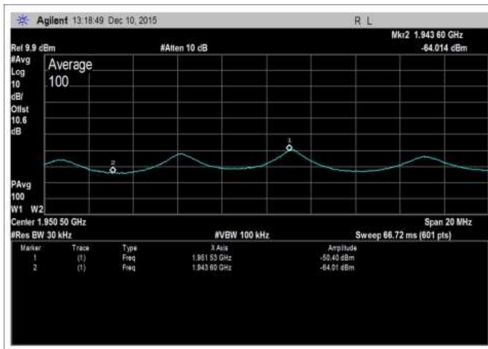
DL-1930-1995-AWG NR+0
