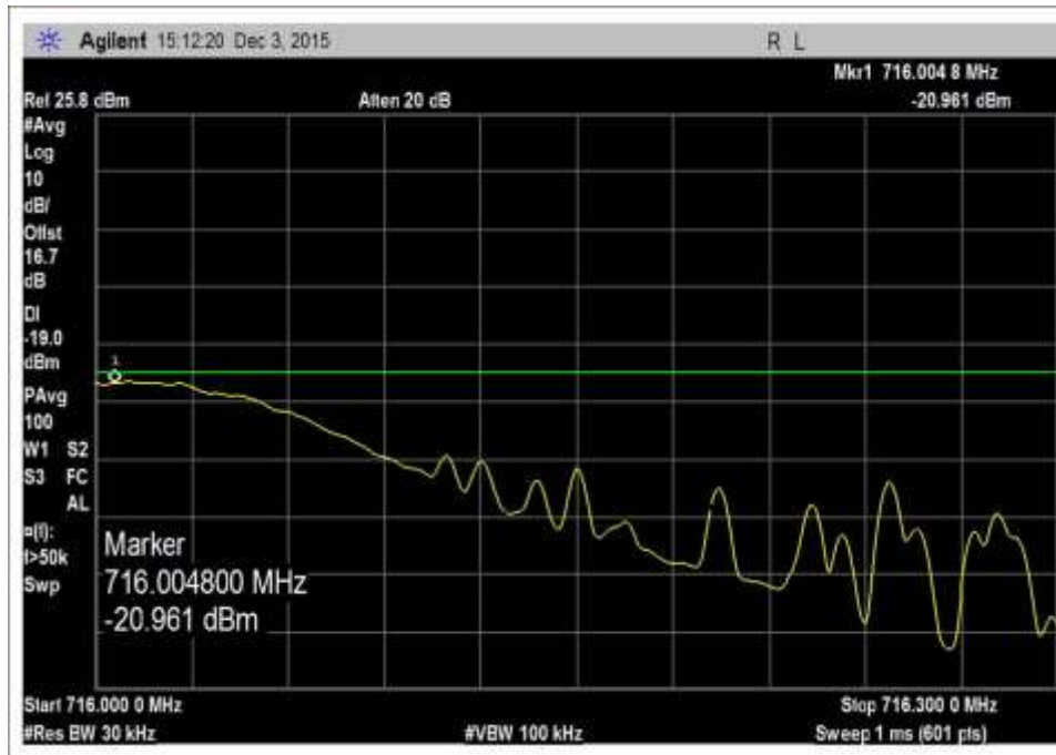
7.5_OBE_UL_698-716MHz_H_0dBm
