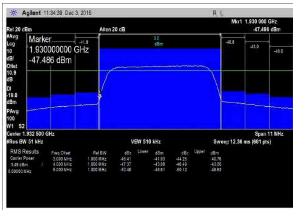
7.5_OBE_DL_1930-1995MHz_L_PreAGC
