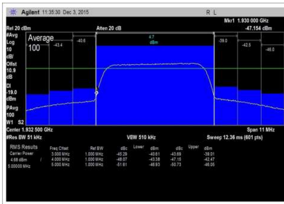
7.5_OBE_DL_1930-1995MHz_L_Max
