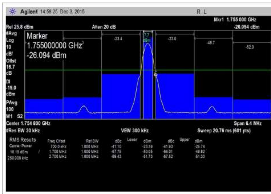
7.5_OBE_UL_1710-1755MHz_H_Max
