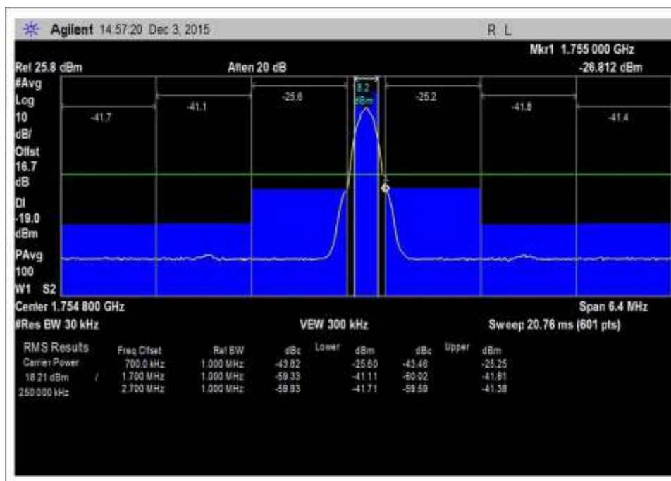
7.5_OBE_UL_1710-1755MHz_H_PreAGC
