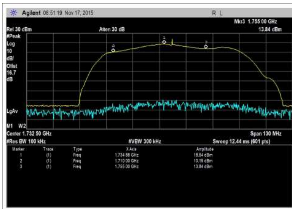
7.1_band verify_UL_1710-1755MHz-Zoom
