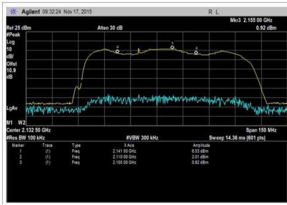
7.1_band verify_DL_2110-2155MHz-Zoom
