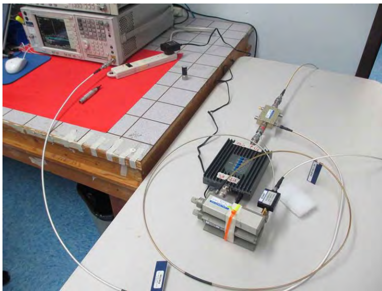
7.7.2 Test Setup
