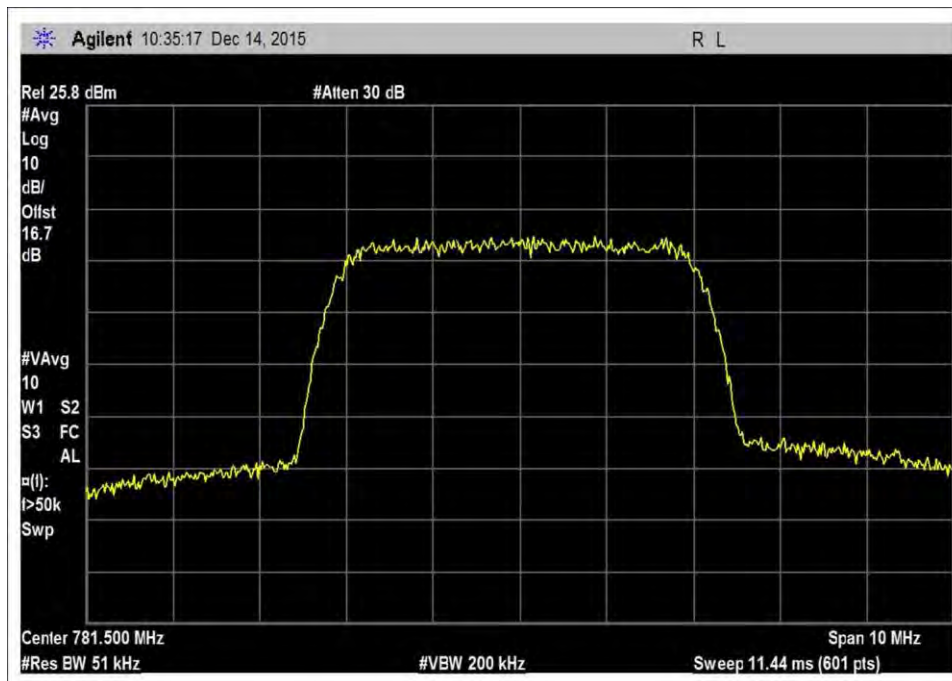
7.10_OBW_UL_776-787MHz_WCDMA
