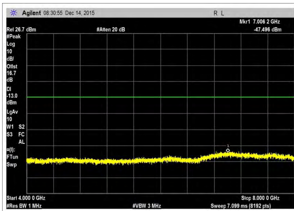
UL_776-787R2
