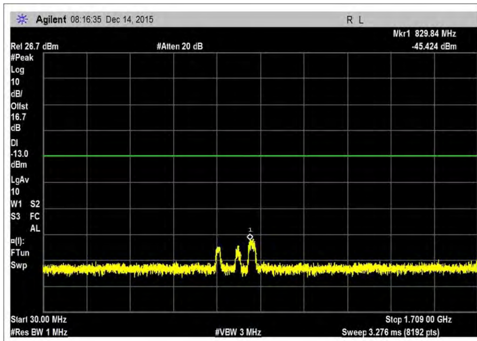
UL_1710-1755L
