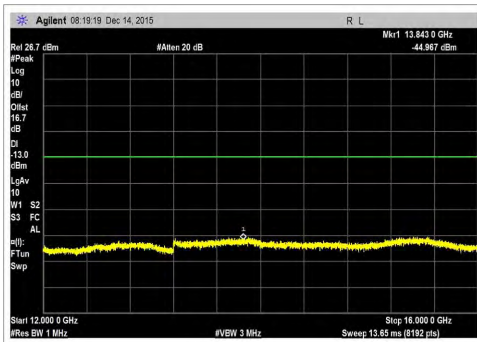
UL_1710-1755R4
