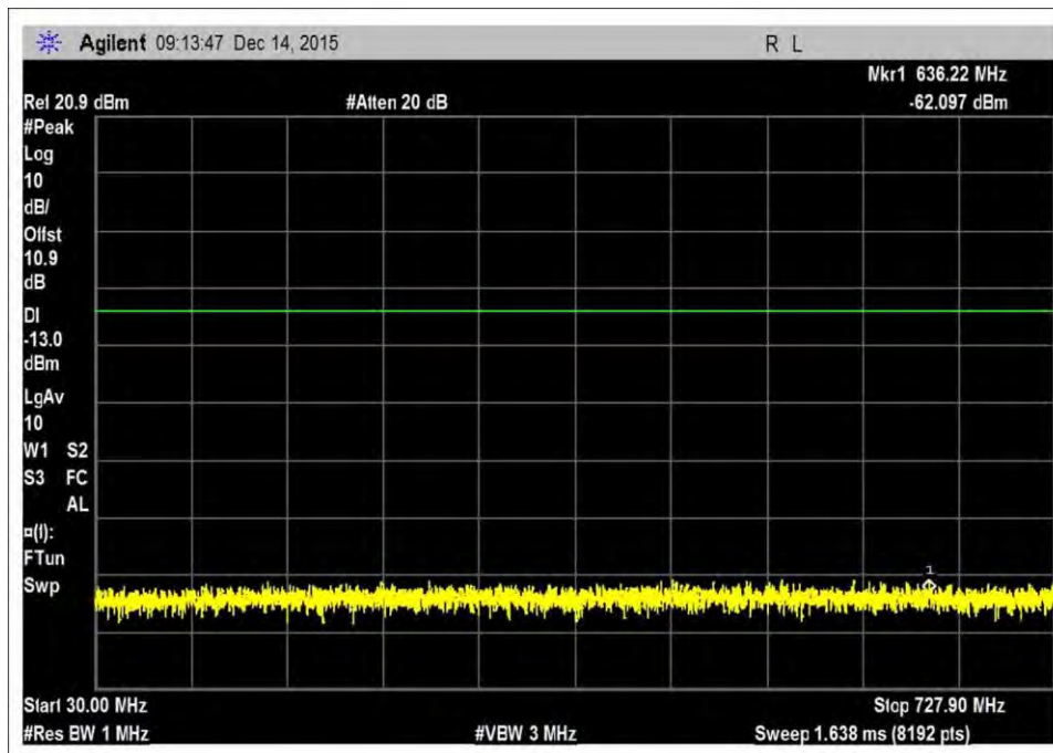
DL_728-746L
