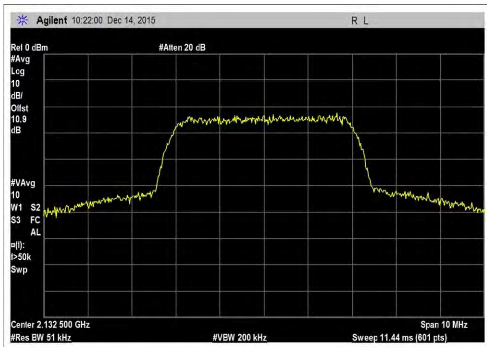
7.10_OBW_DL_2110-2155MHz_WCDMA
