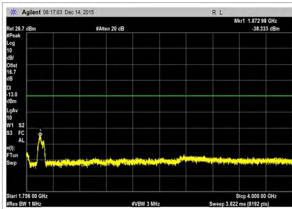
UL_1710-1755R1
