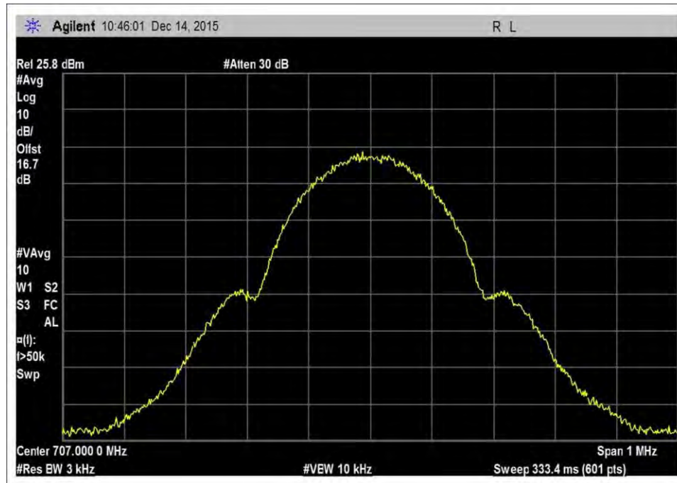
7.10_OBW_UL_698-716MHz_GSM
